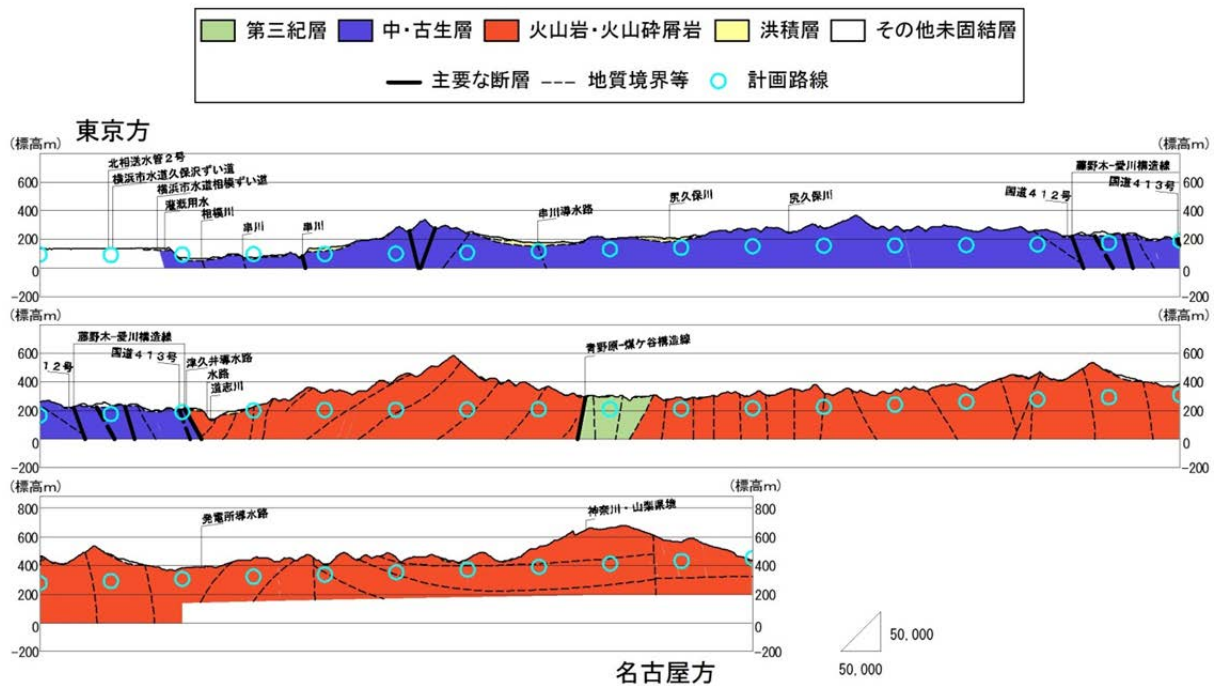
図 8-2-3-12 地質縦断図
