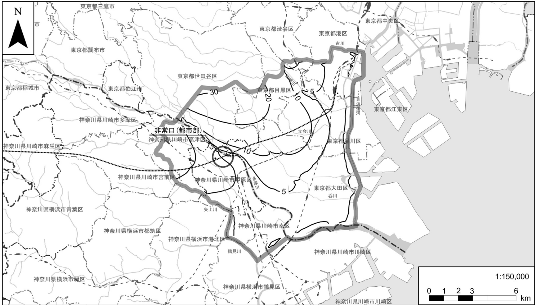
凡例 ..... 計画路線(トンネル部) 解析範囲 - - - 都県境 地下水位等高線(標高m) - - - 区市境 図8-2-3-15(1) 水位等高線図(浅層) [構造物を考慮した場合]
