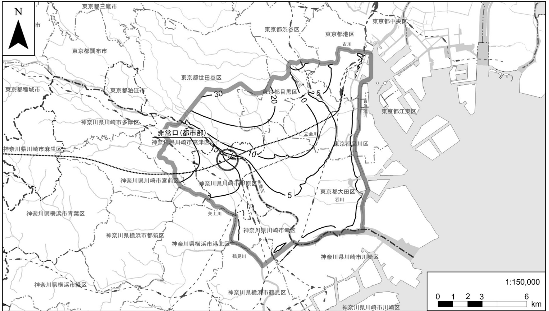
凡例 ..... 計画路線(トンネル部) 解析範囲 - - - 都県境 地下水位等高線(標高m) - · - · 区市境 図8-2-3-14(1) 水位等高線図(浅層) [構造物を考慮しない場合(現況)]
