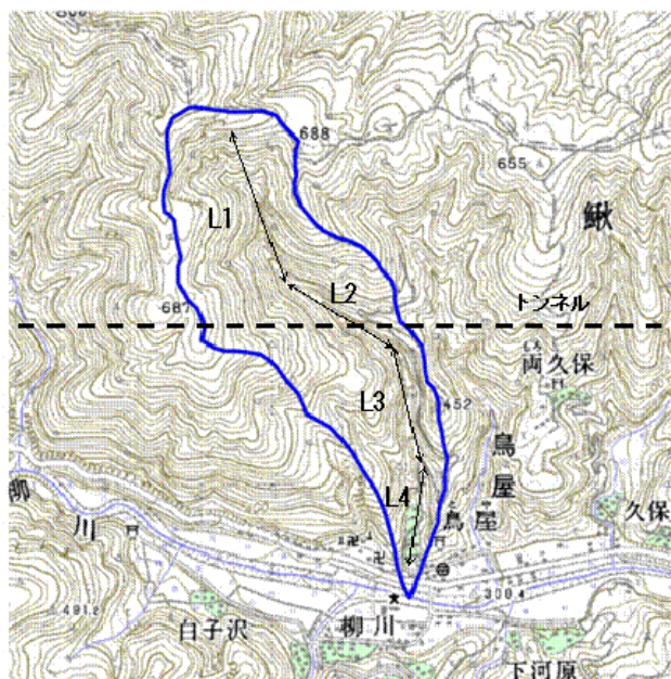
図 7-2-1-1 単位流域及び流路延長の設定概要
