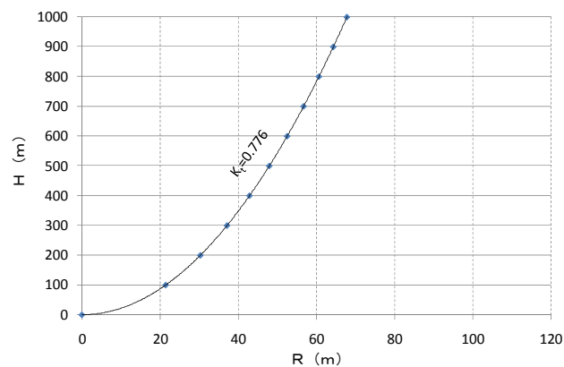
図 7-2-5-1 H-R 曲線の概要
