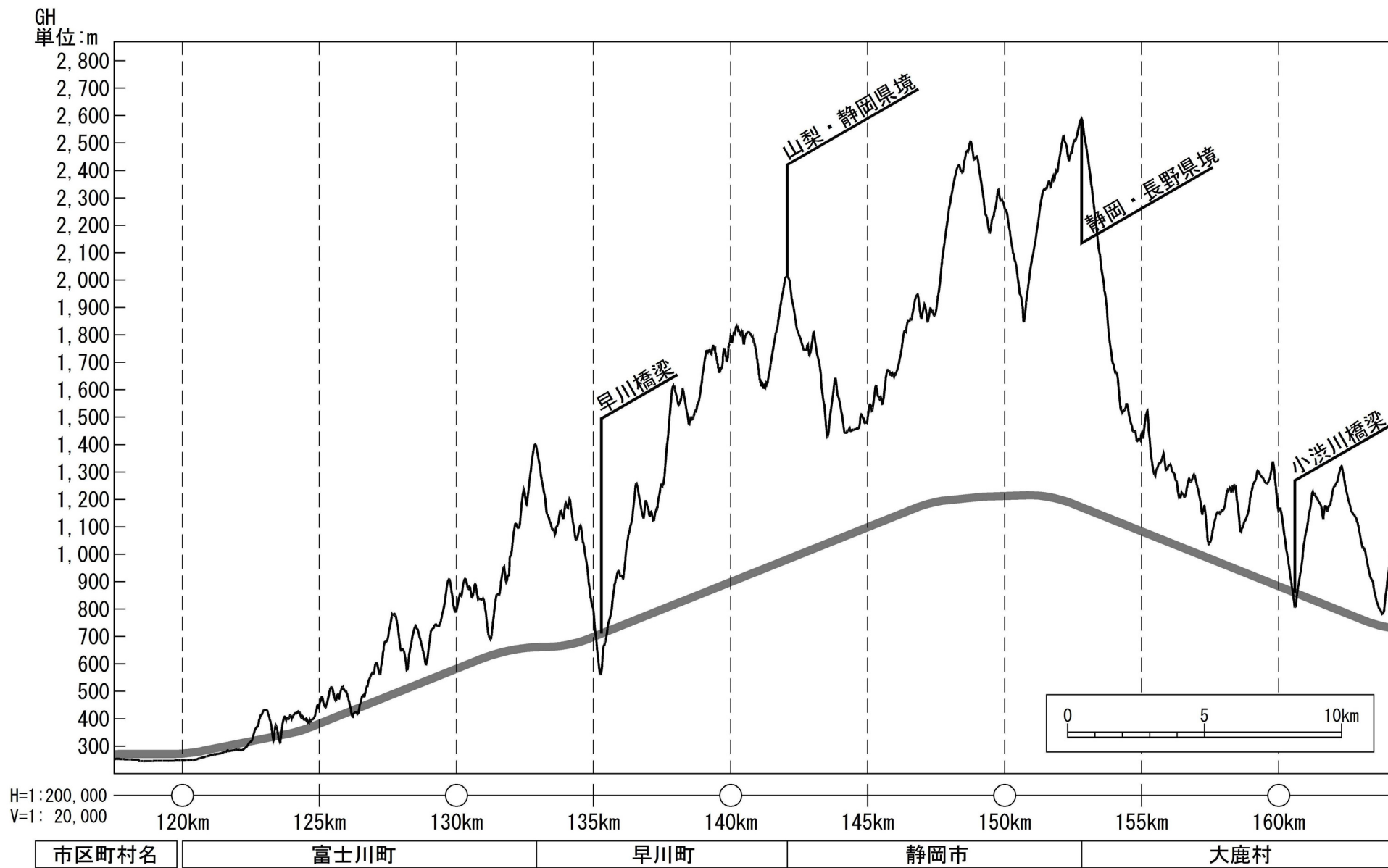
図 2-1(4) 路線概要 (縦断計画)
