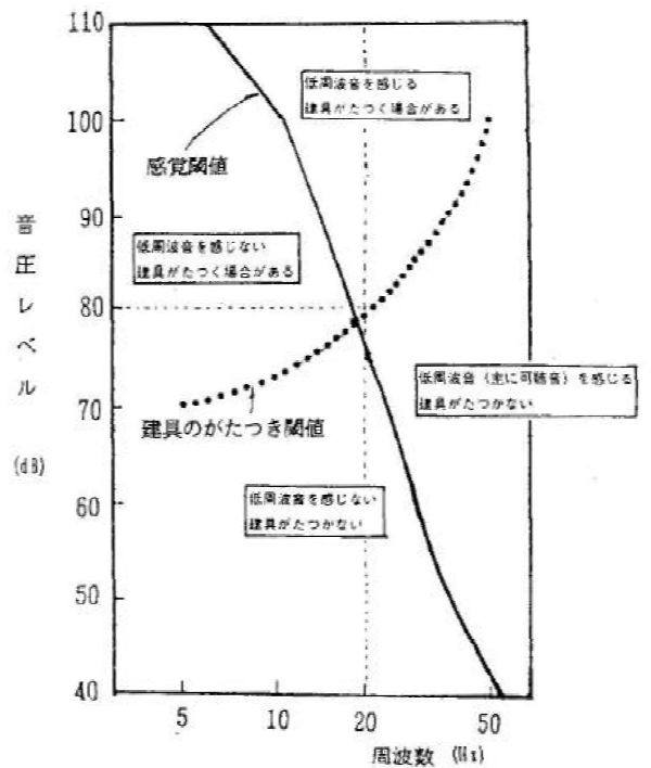
図 8-1-5-5 建具等のがたつきの閾値
