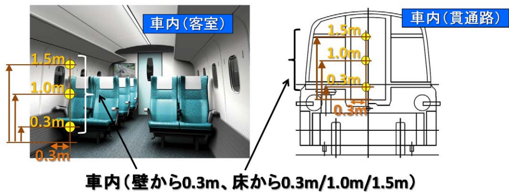
図 12-5-3 車内の磁界の測定箇所
