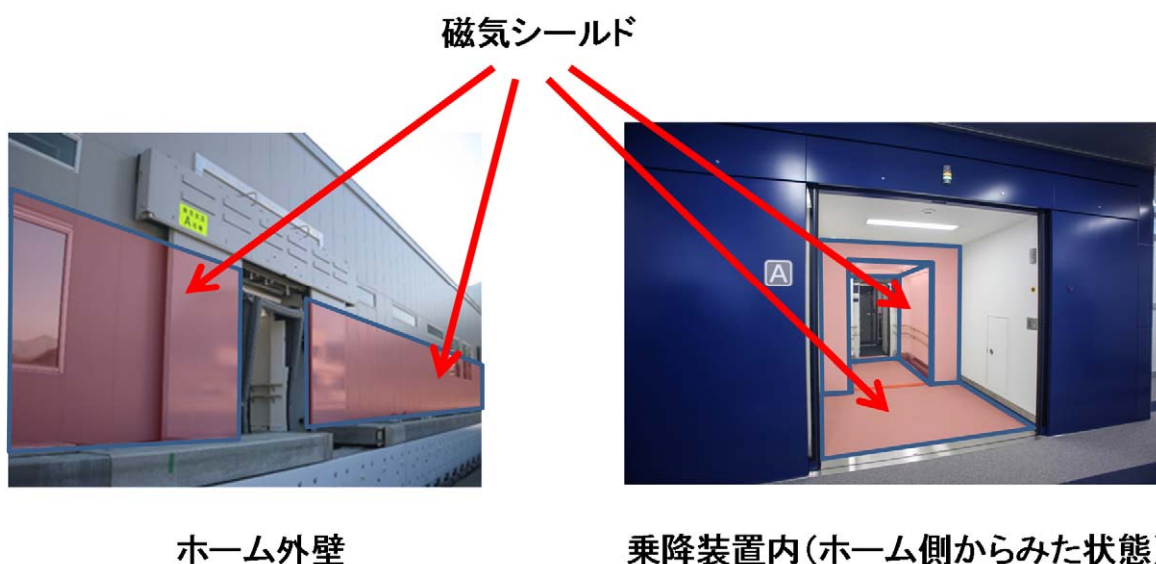
図 12-5-2 ホームへの磁気シールド設置の概念図
