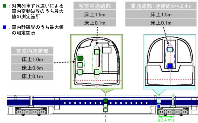
図 12-5-6 車内の磁界の測定箇所
