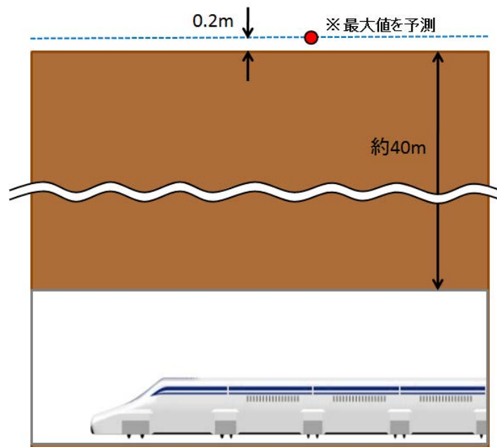
図 12-7-3-2 地上における磁界の算出位置イメージ（ケース 2）
