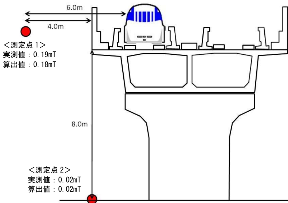
図 12-7-2-1 山梨リニア実験線における実測値と算出値の比較
