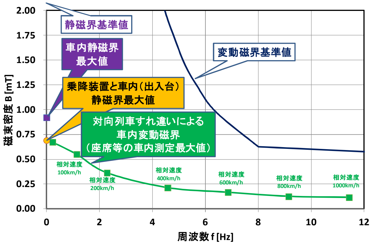
図 12-5-5 車内及び乗降装置と車内（出入台）の磁界の測定結果
