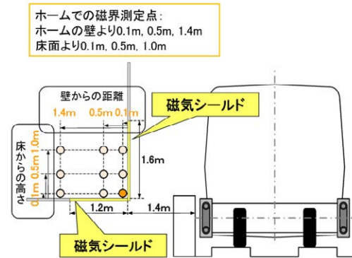
図 12-5-7 ホーム上の磁界の測定箇所
