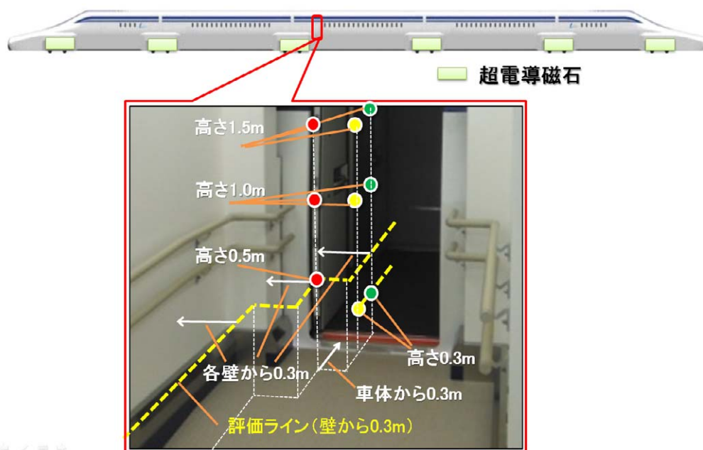
図 12-5-4 乗降装置と車内(出入台)の磁界の測定箇所
