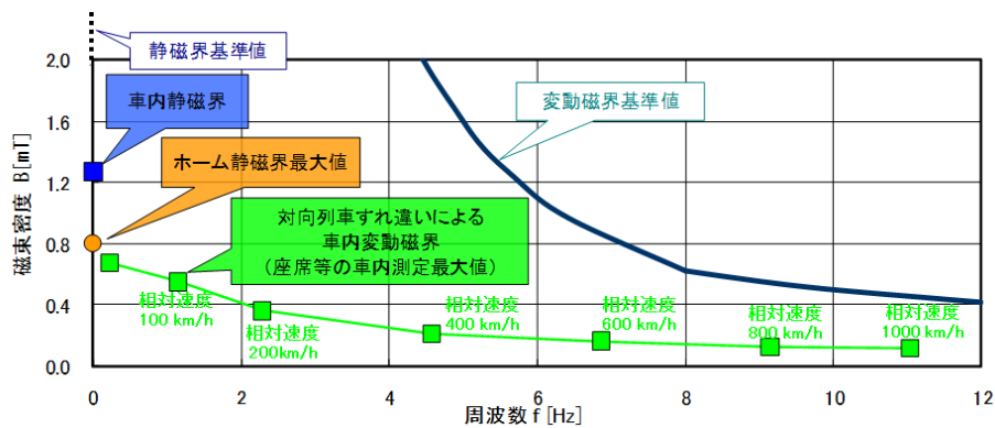
図 12-5-8 車内及びホームの磁界の測定結果
