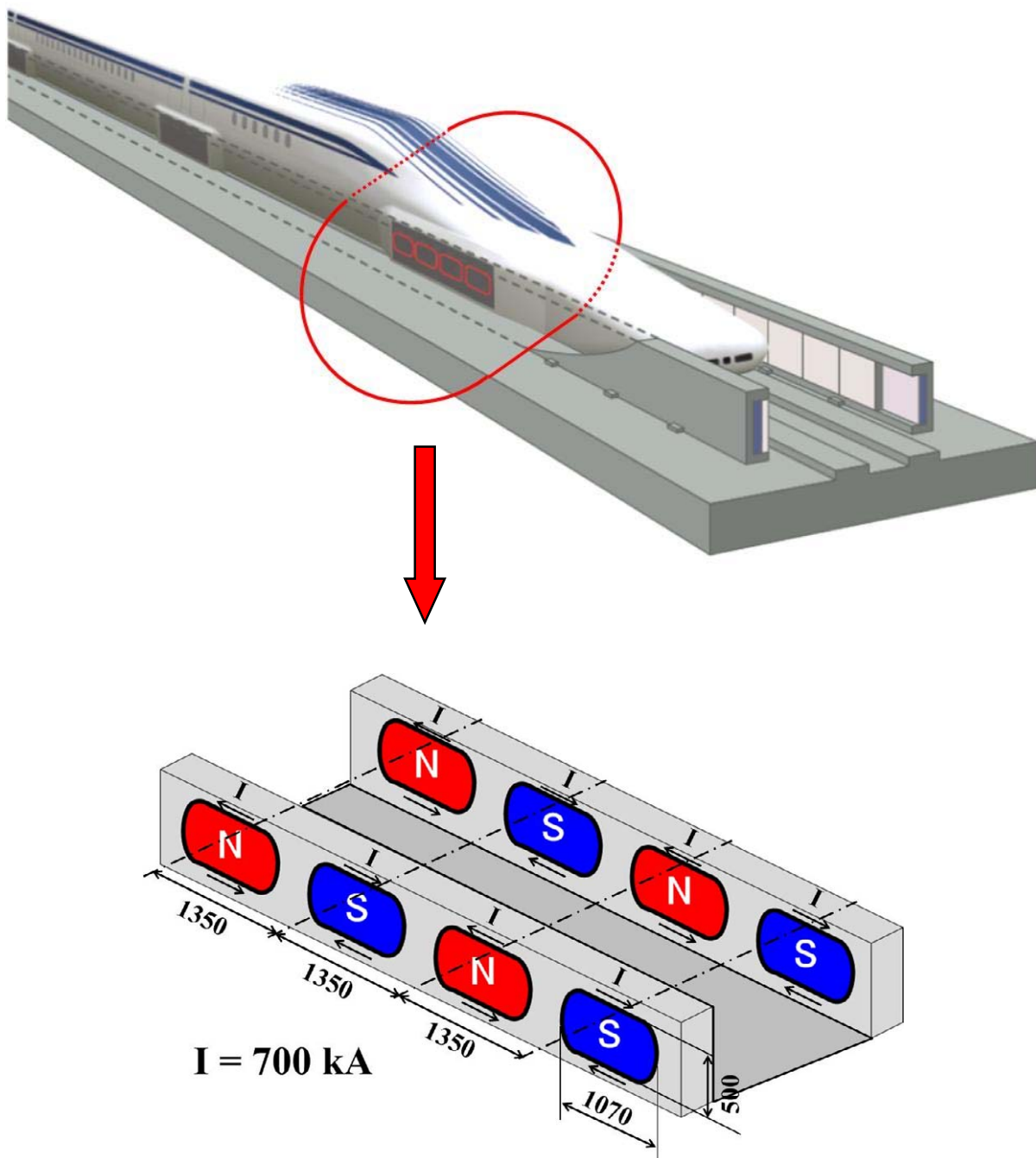
図 12-7-1-2 超電導磁石を拡大した概略図（磁界の算出にあたっての前提条件）
