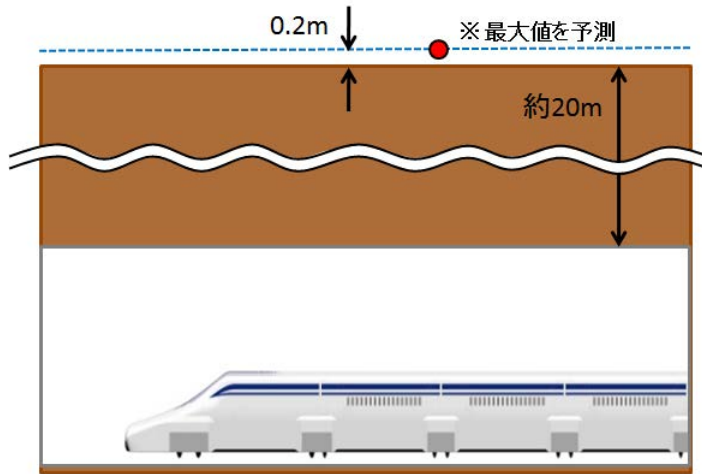
図 12-7-3-1 地上における磁界の算出位置イメージ（ケース 1）
