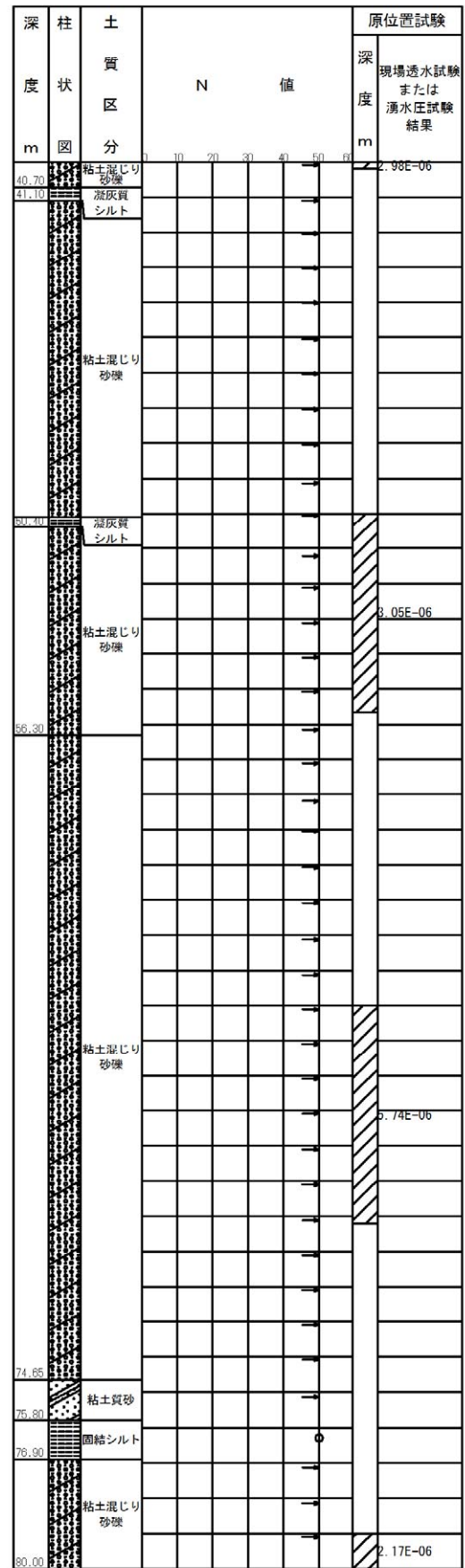
図 6-4-1-2(1) ボーリング柱状図 (地点 01-1)
