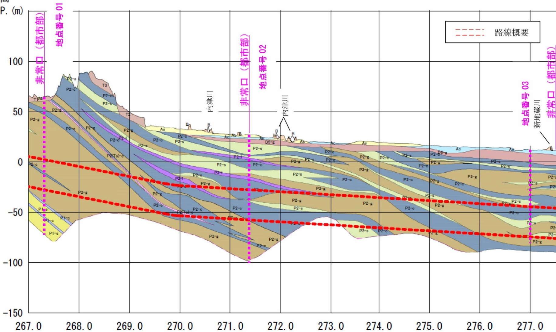
図 6-4-2-1(1) 都市トンネル区間縦断面図 (春日井市)
