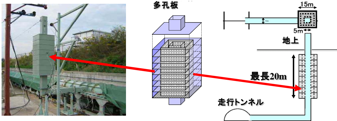
図 4-2-3-1 模擬模型試験イメージ
