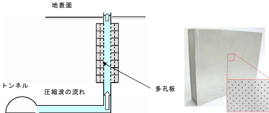
図 4-3-2-1 多孔板の構造
