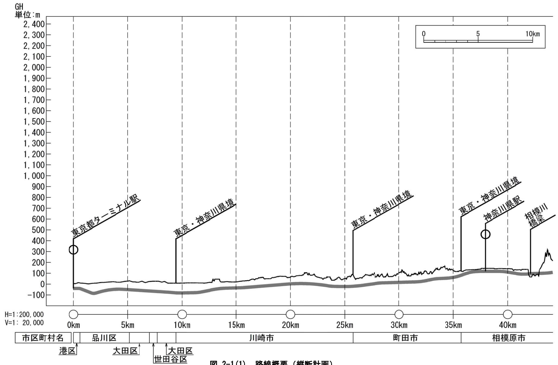
図 2-1(1) 路線概要 (縦断計画)
