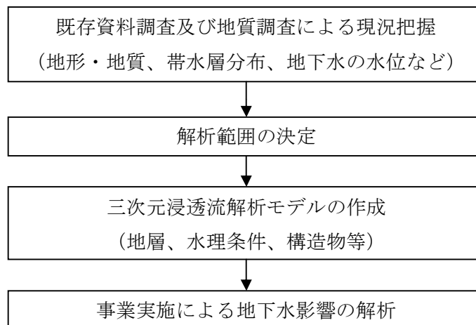
図 8-2-2-3 三次元浸透流解析による予測手順
