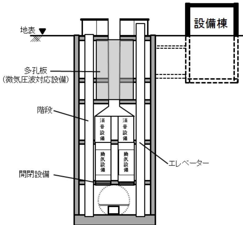
図 3-4-6-5 都市部における換気施設（非常口）の概要
