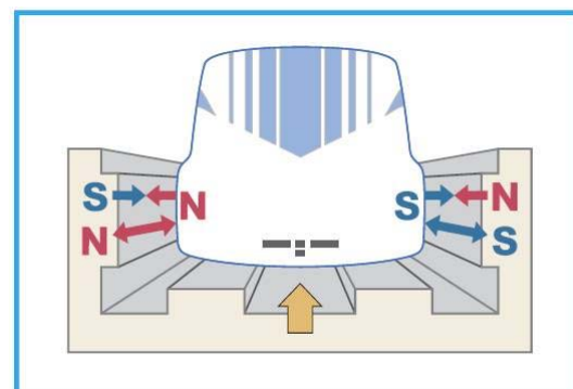
図 3-4-10-4 浮上の原理
