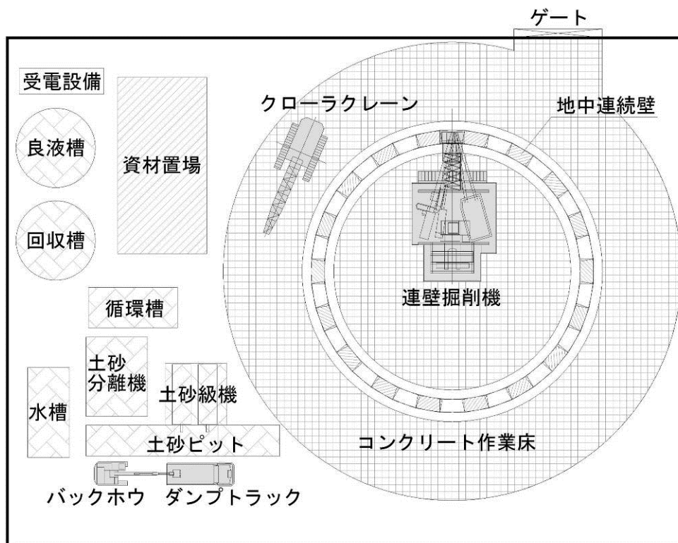
図 3-4-6-19 非常口の施工ヤードの概要（RC地中連続壁工法による非常口施工時）
