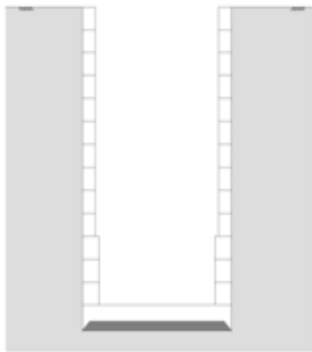
図 3-4-6-18 非常口の施工概要 (ケーソン工法の場合)
