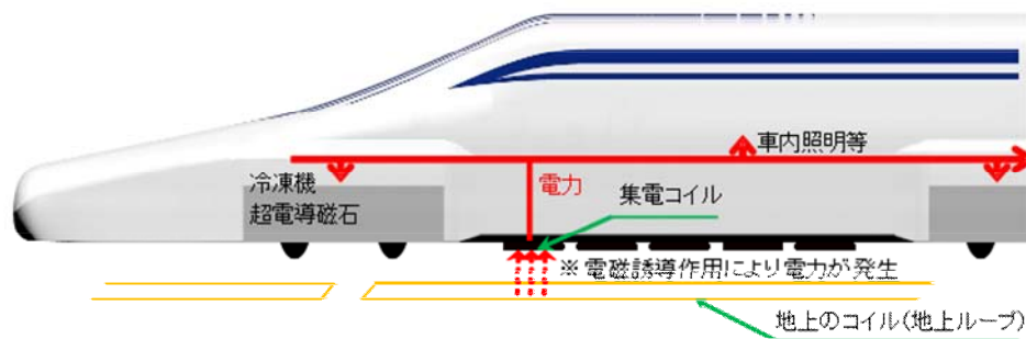
図 3-4-10-7 車上電源供給の概要
