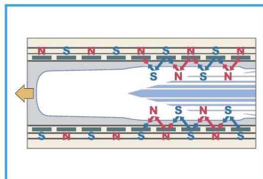
図 3-4-10-3 推進の原理
