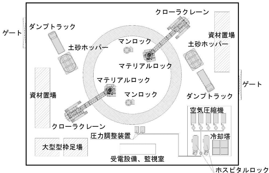
図 3-4-6-20 非常口の施工ヤードの概要（ケーソン工法による非常口施工時）
