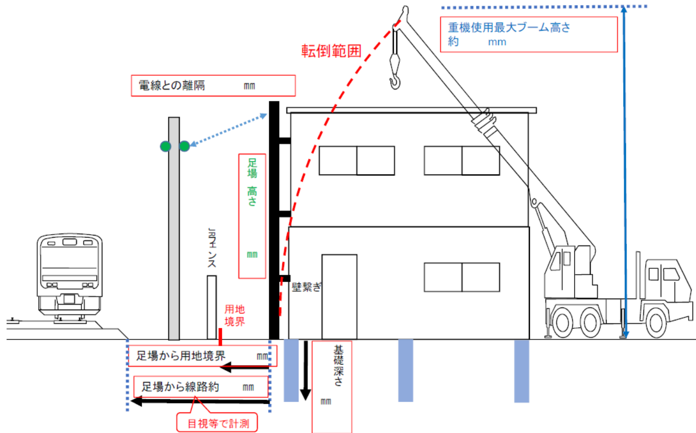
断面図
