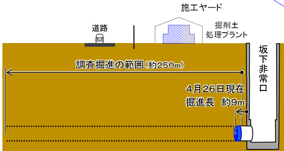
坂下非常口付近の断面図
