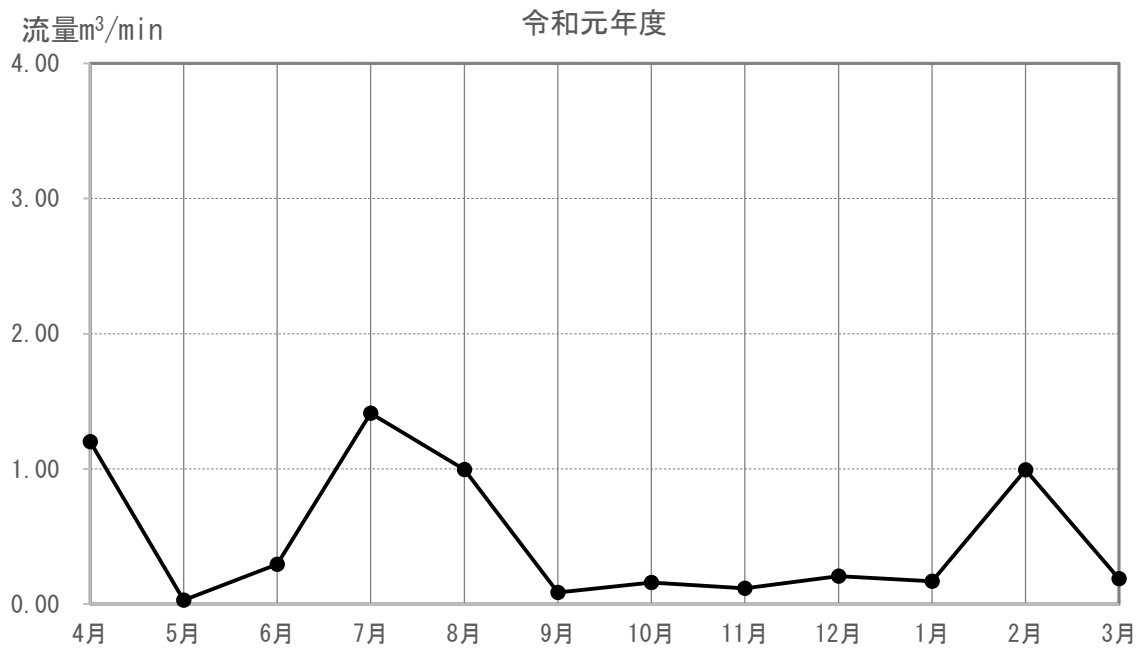
図 3-5-4-2 (57) 河川の流量の調査結果 (M-115)
