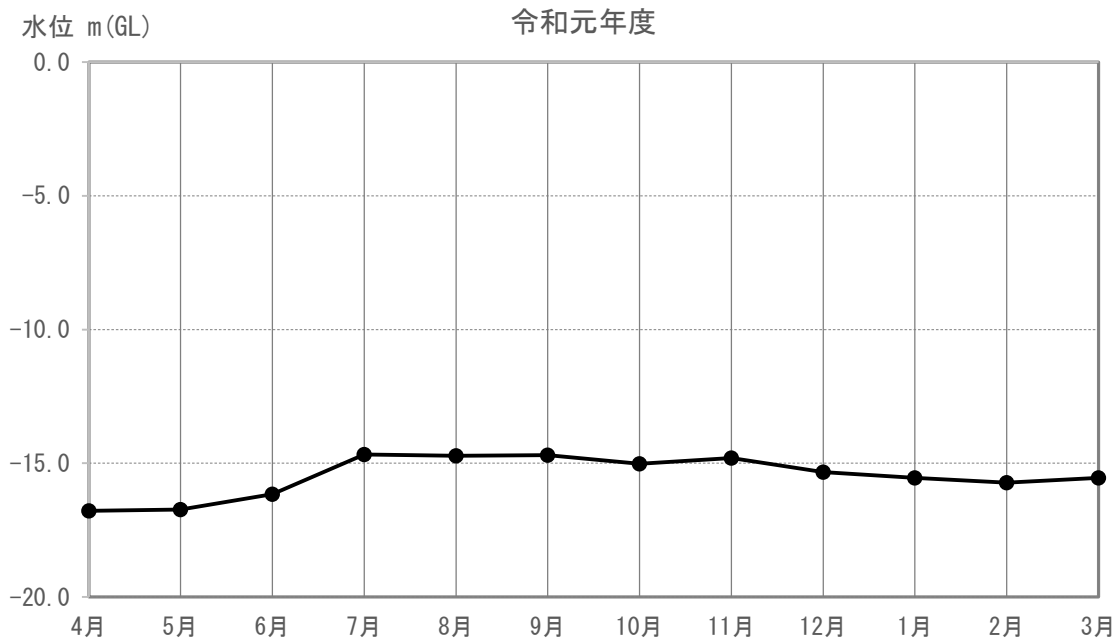
図 3-5-4-1(63) 地下水の水位（又は水量）の調査結果(T-102)
