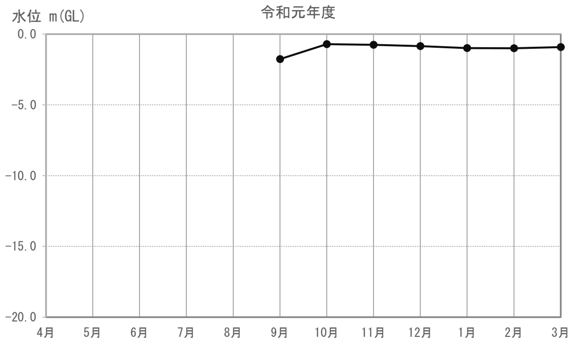
図 3-5-4-1(21) 地下水の水位（又は水量）の調査結果(N-134)
