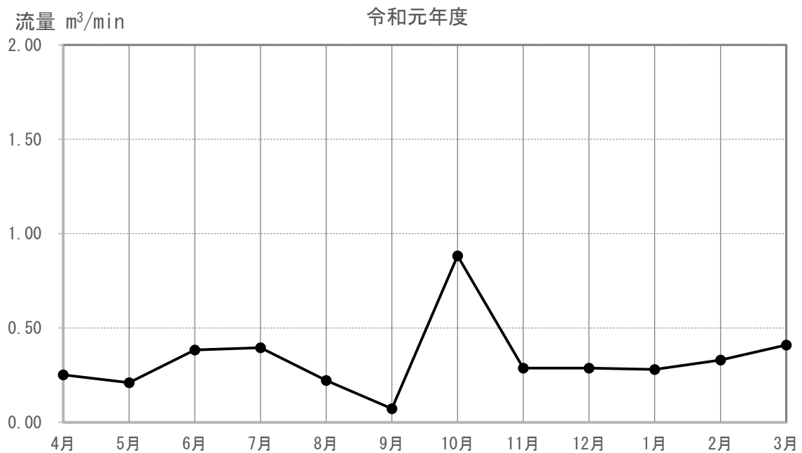
図 3-5-4-2(90) 河川の流量の調査結果(M-147)
