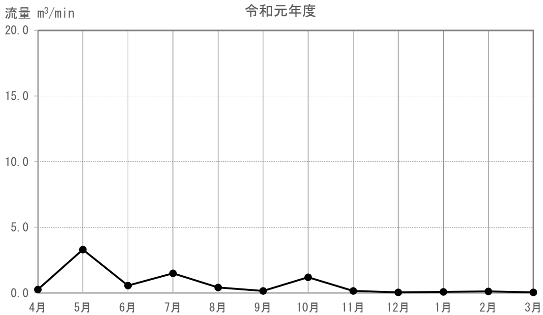
図 3-5-4-2(130) 河川の流量の調査結果(T-118)
