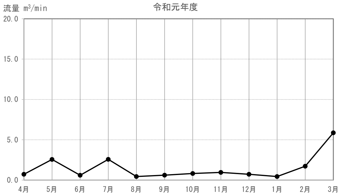
図 3-5-4-2 (55) 河川の流量の調査結果 (E-139)
