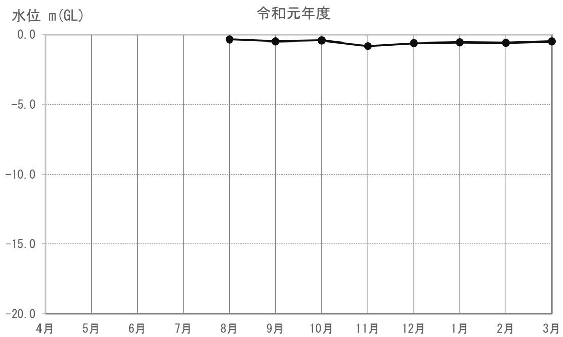
図 3-5-4-1(28) 地下水の水位（又は水量）の調査結果(N-141)
