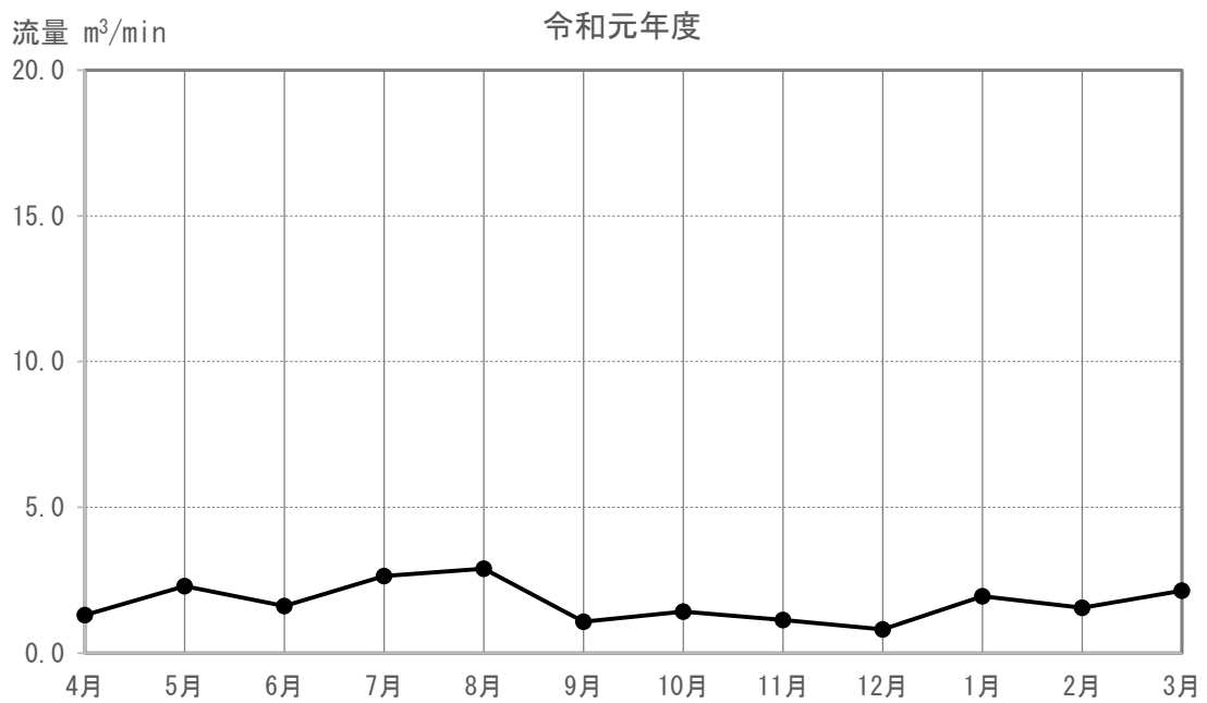
図 3-5-4-2(104) 河川の流量の調査結果(K-110)
