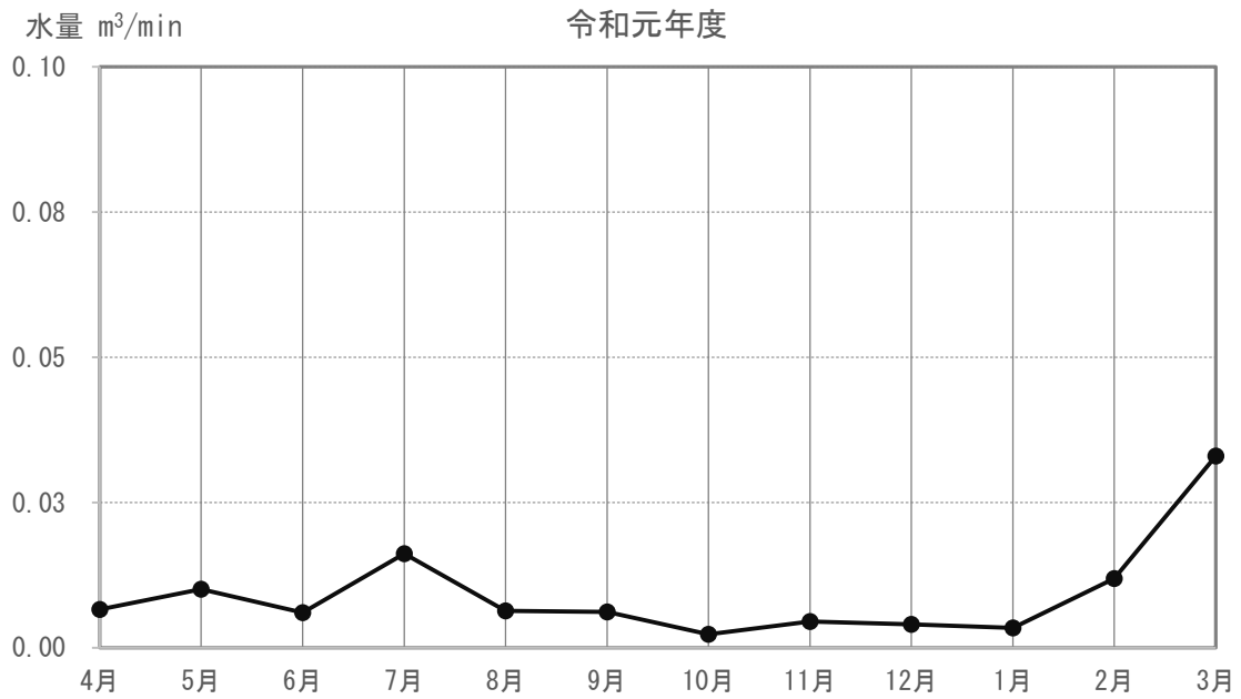
図 3-5-4-1(39) 地下水の水位（又は水量）の調査結果(E-110)
