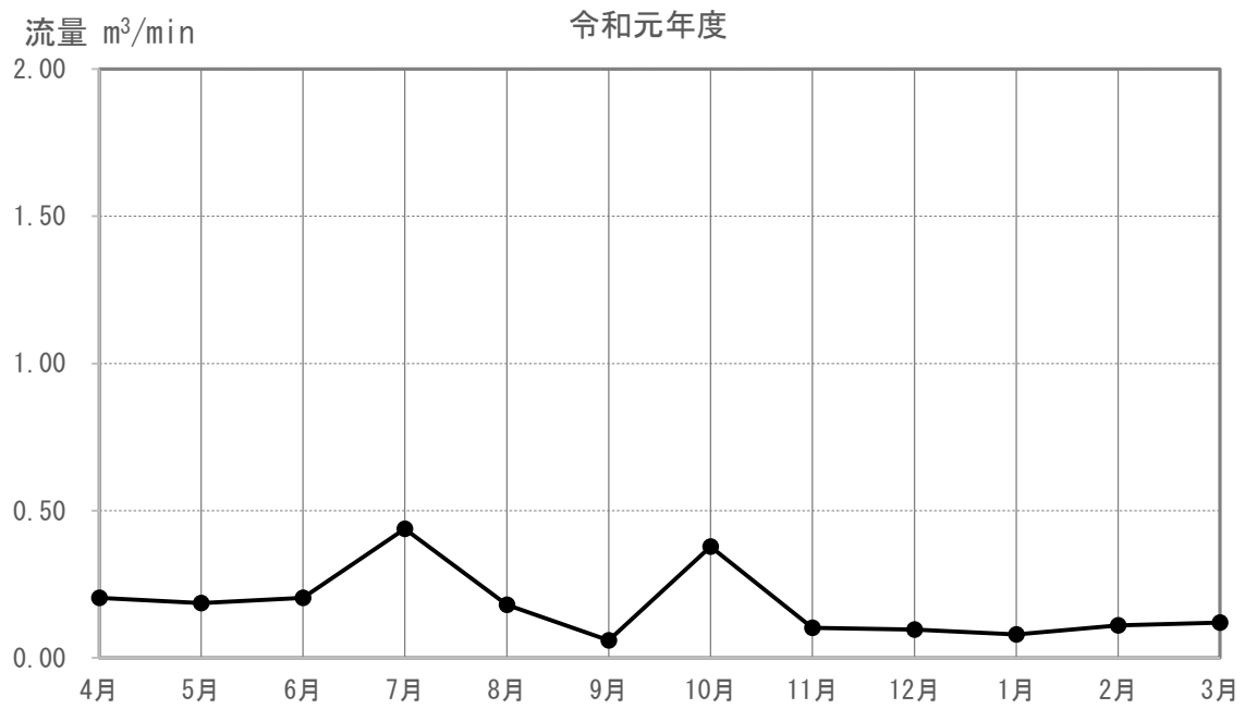
図 3-5-4-2(77) 河川の流量の調査結果(M-134)
