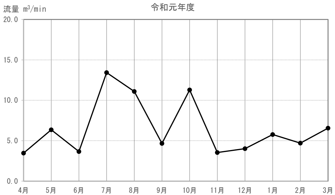
図 3-5-4-2(114) 河川の流量の調査結果 (K-120)
