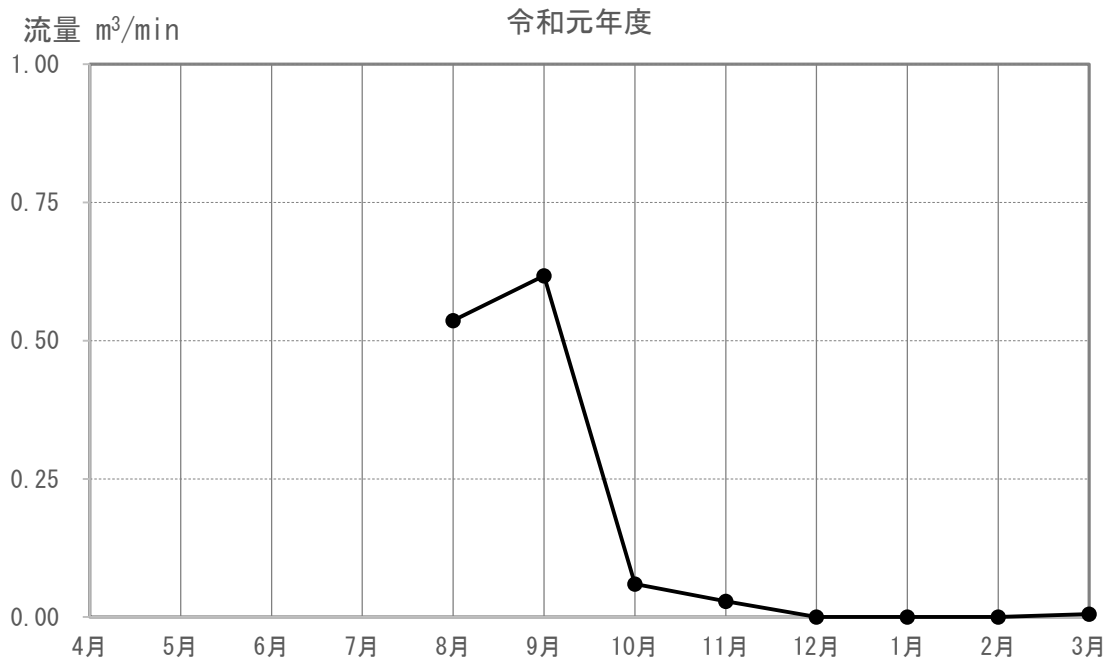
図 3-5-4-2(22) 河川の流量の調査結果 (N-151)
