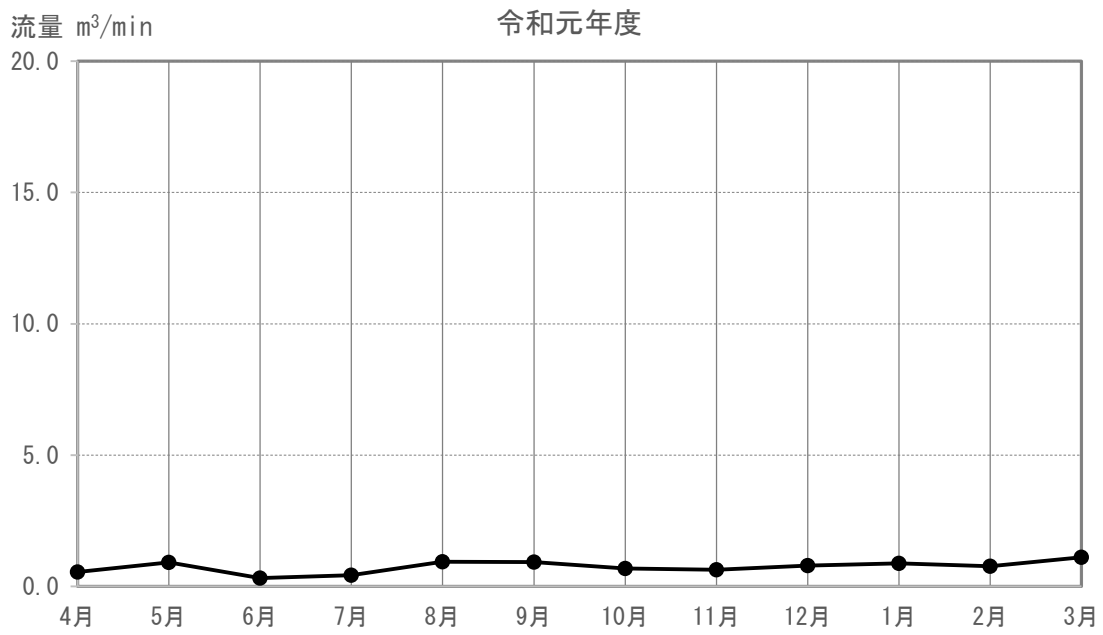
図 3-5-4-2 (49) 河川の流量の調査結果 (E-133)
