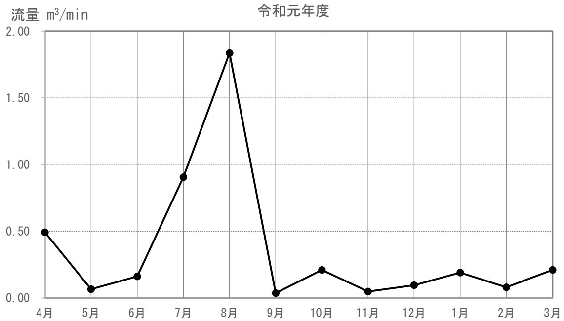
図 3-5-4-2(64) 河川の流量の調査結果(M-121)
