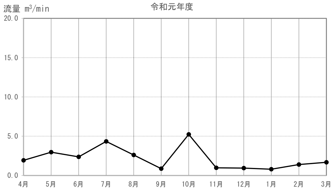
図 3-5-4-2 (81) 河川の流量の調査結果 (M-138)
