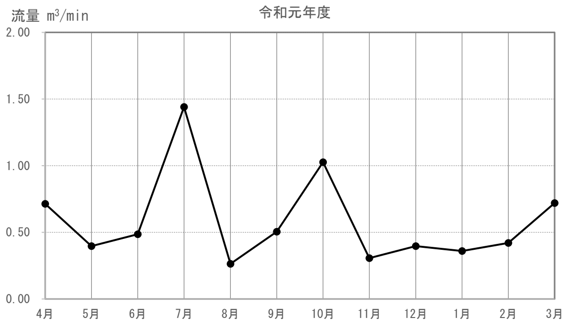
図 3-5-4-2(78) 河川の流量の調査結果(M-135)
