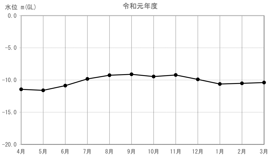
図 3-5-4-1 (62) 地下水の水位（又は水量）の調査結果 (T-101)
