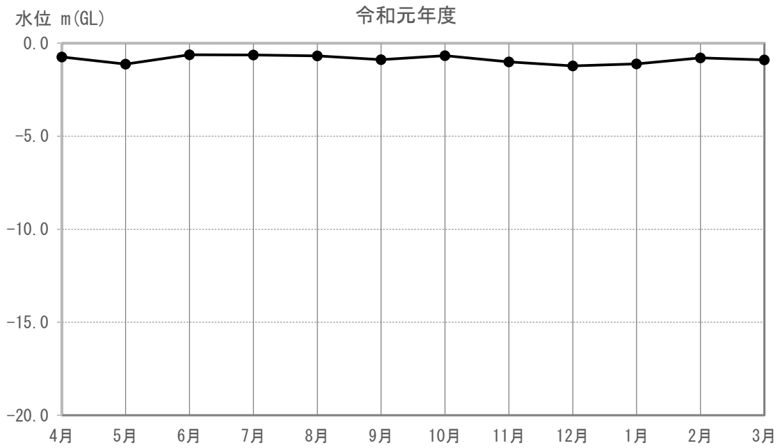
図 3-5-4-1 (65) 地下水の水位（又は水量）の調査結果 (T-104)
