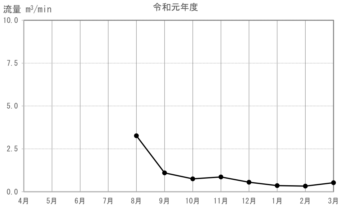
図 3-5-4-2(21) 河川の流量の調査結果 (N-150)
