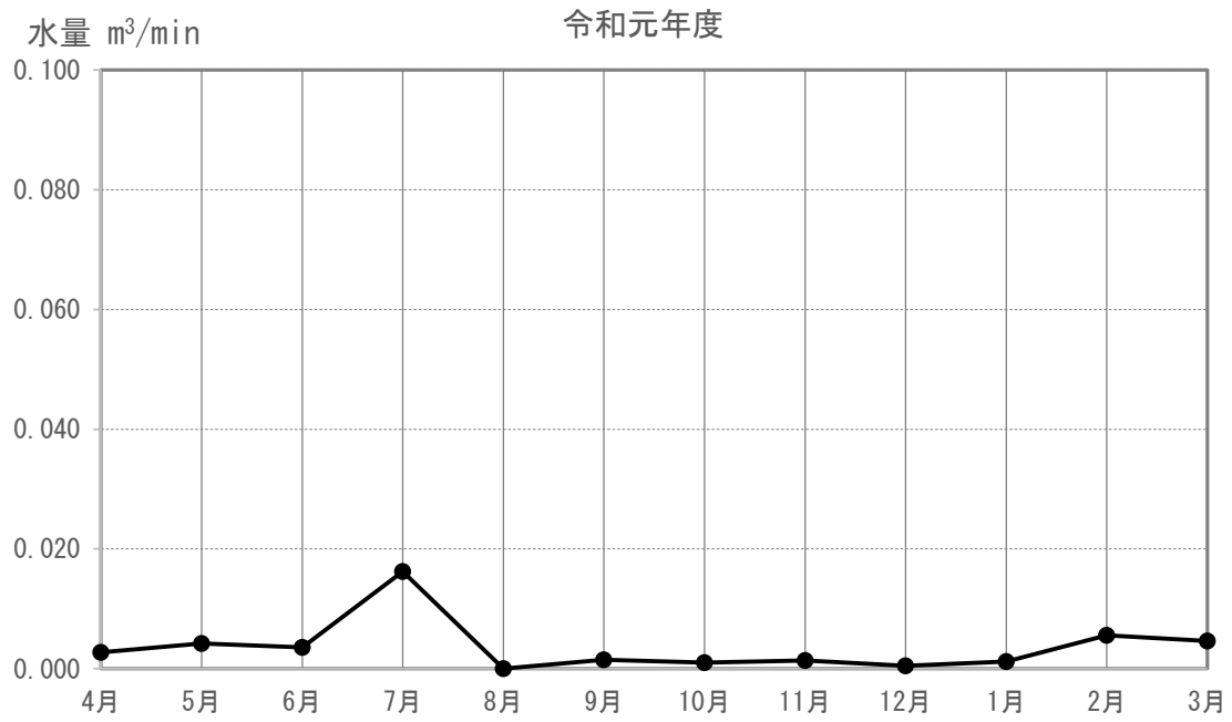
図 3-5-4-1(47) 地下水の水位（又は水量）の調査結果(M-157)
