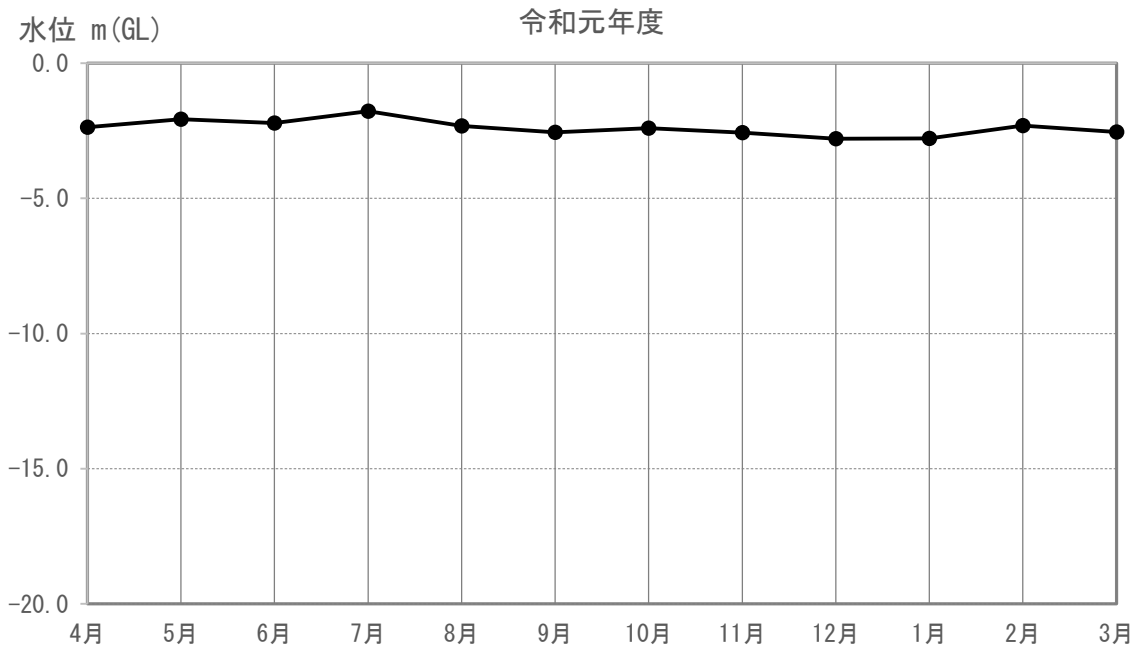
図 3-5-4-1(49) 地下水の水位（又は水量）の調査結果(M-107)
