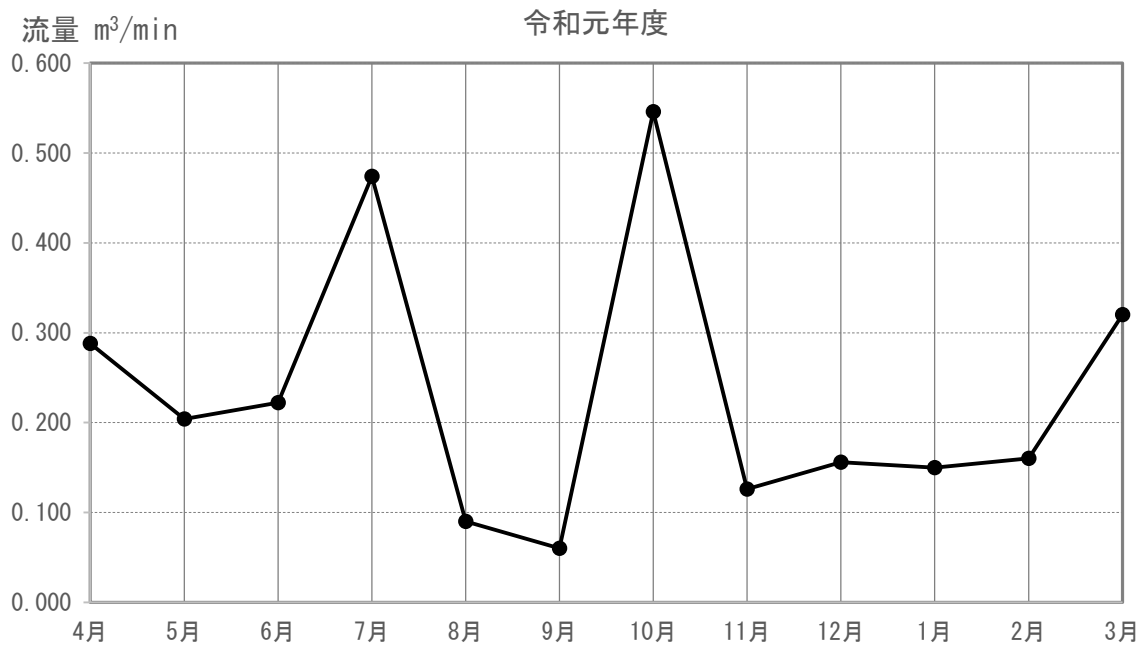
図 3-5-4-2 (91) 河川の流量の調査結果 (M-148)
