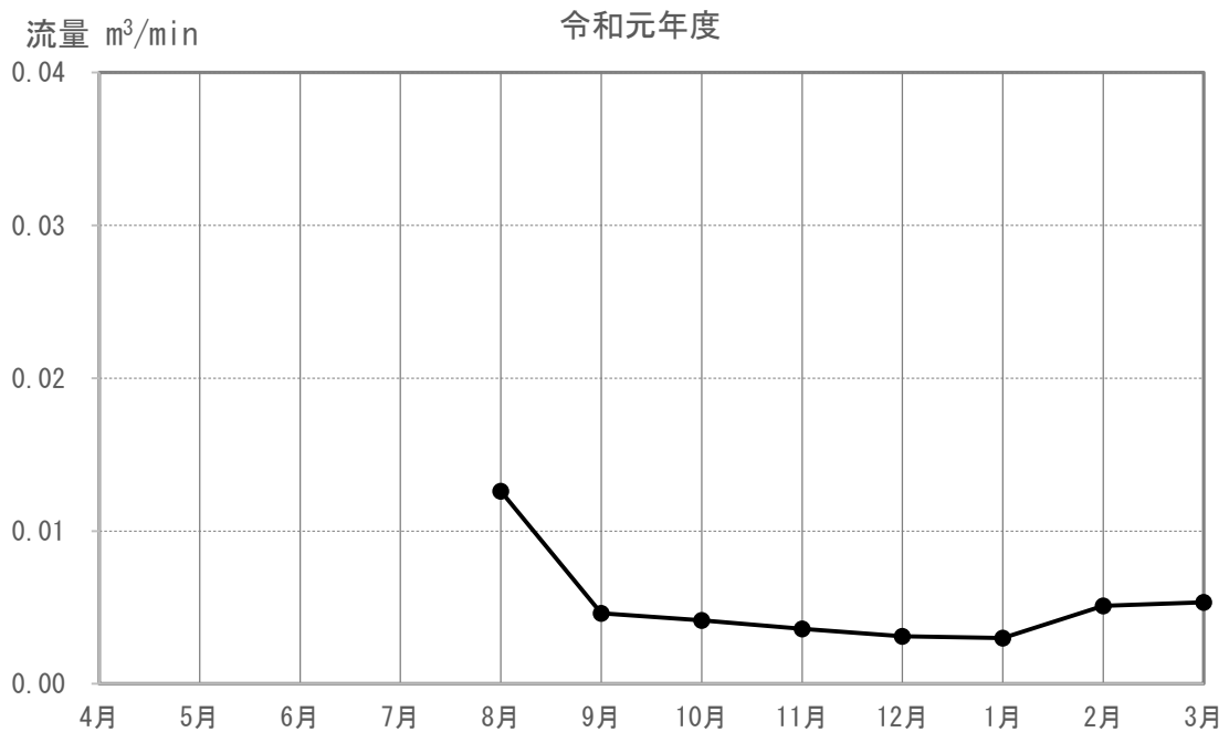
図 3-5-4-2 (26) 河川の流量の調査結果 (N-155)
