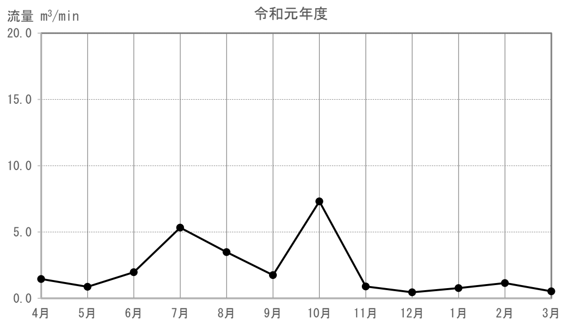
図 3-5-4-2(127) 河川の流量の調査結果(T-115)
