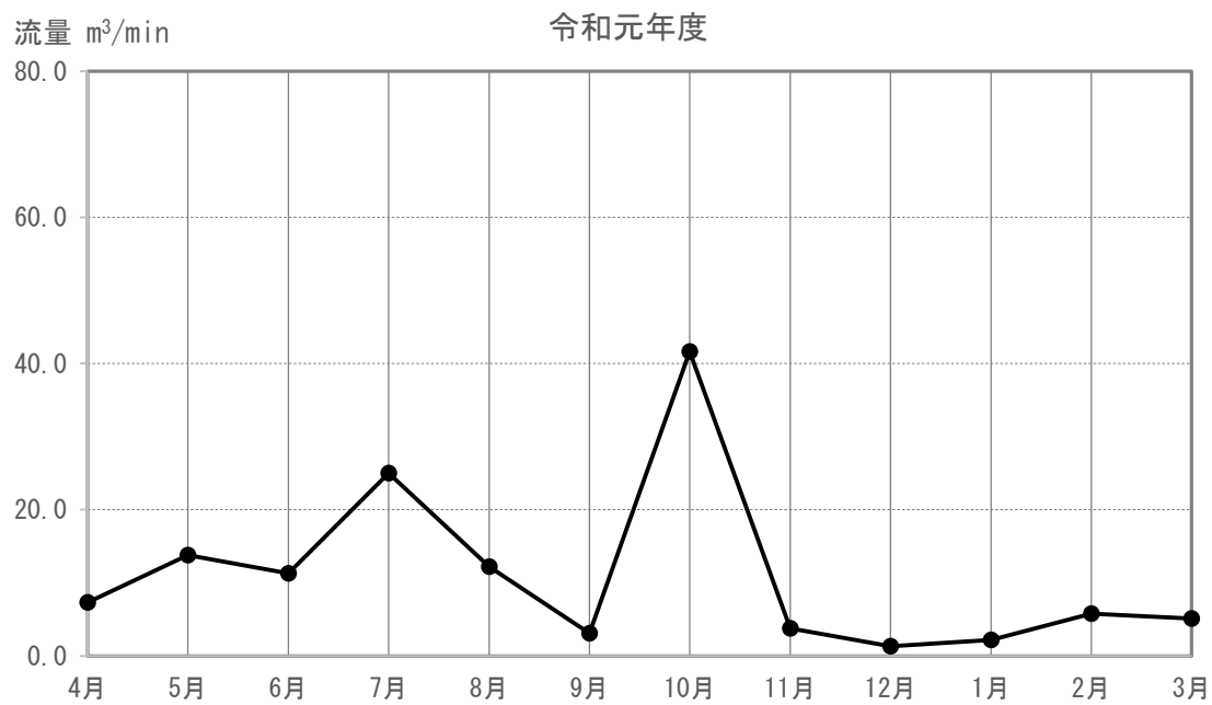
図 3-5-4-2(135) 河川の流量の調査結果(T-123)
