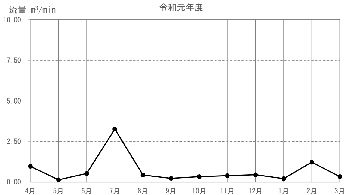
図 3-5-4-2 (59) 河川の流量の調査結果 (M-117)
