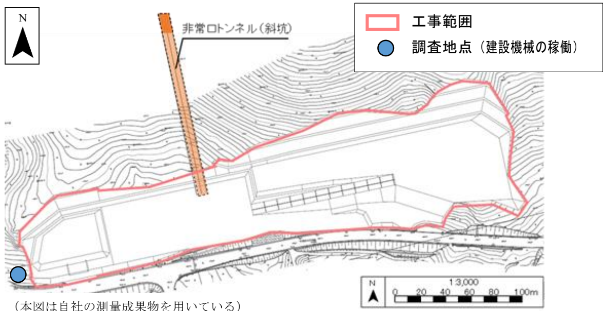
図 3-2-3-1(2) 工事最盛期のモニタリングの実施地点（騒音）（02 瀬戸）
