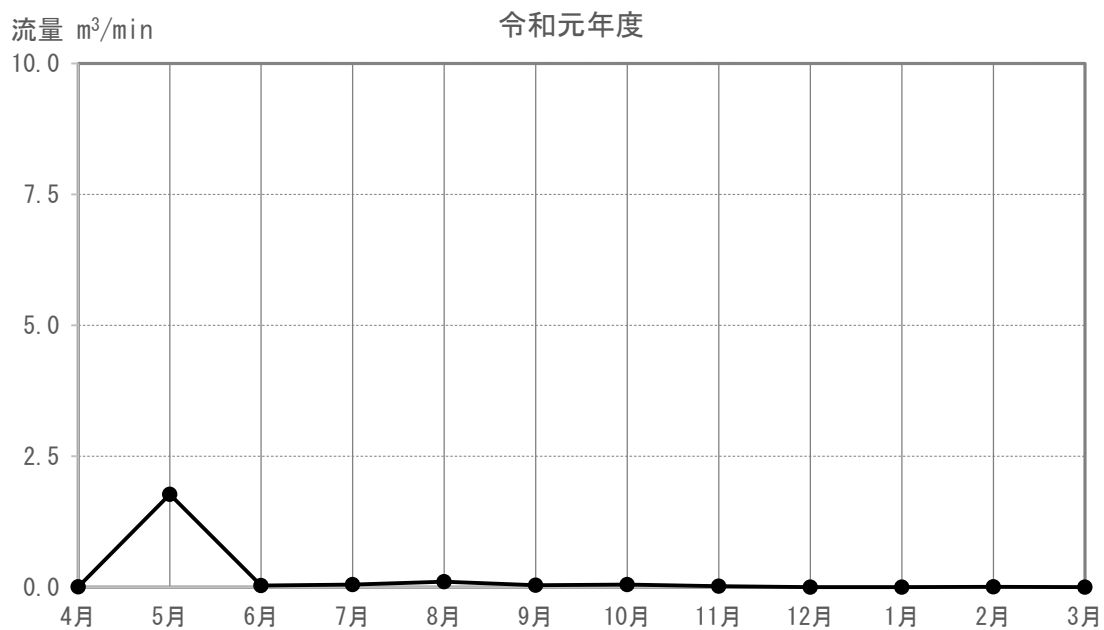
図 3-5-4-2(125) 河川の流量の調査結果(T-113)
