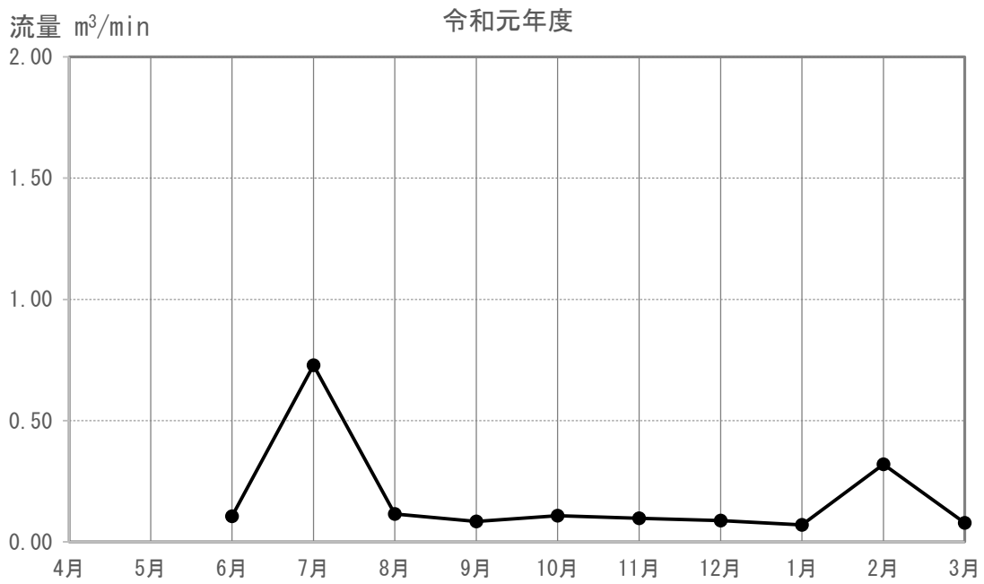
図 3-5-4-2(61) 河川の流量の調査結果(M-159)
