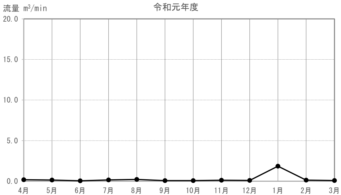
図 3-5-4-2 (34) 河川の流量の調査結果(E-118)
