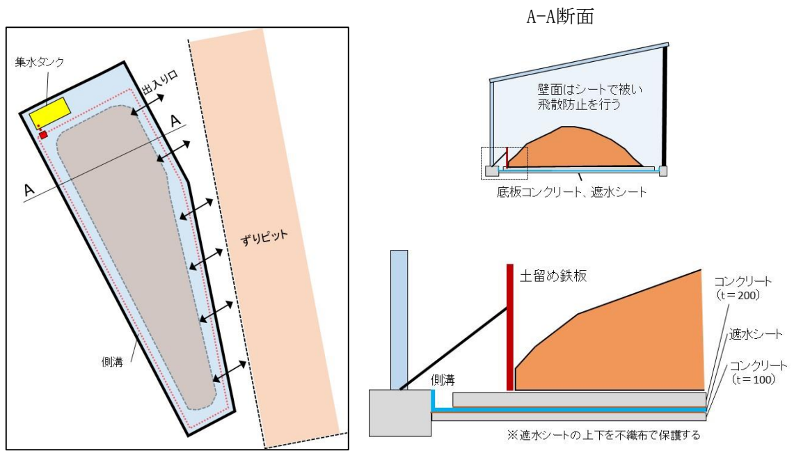
図 参-3-2 スtockヤード構造
