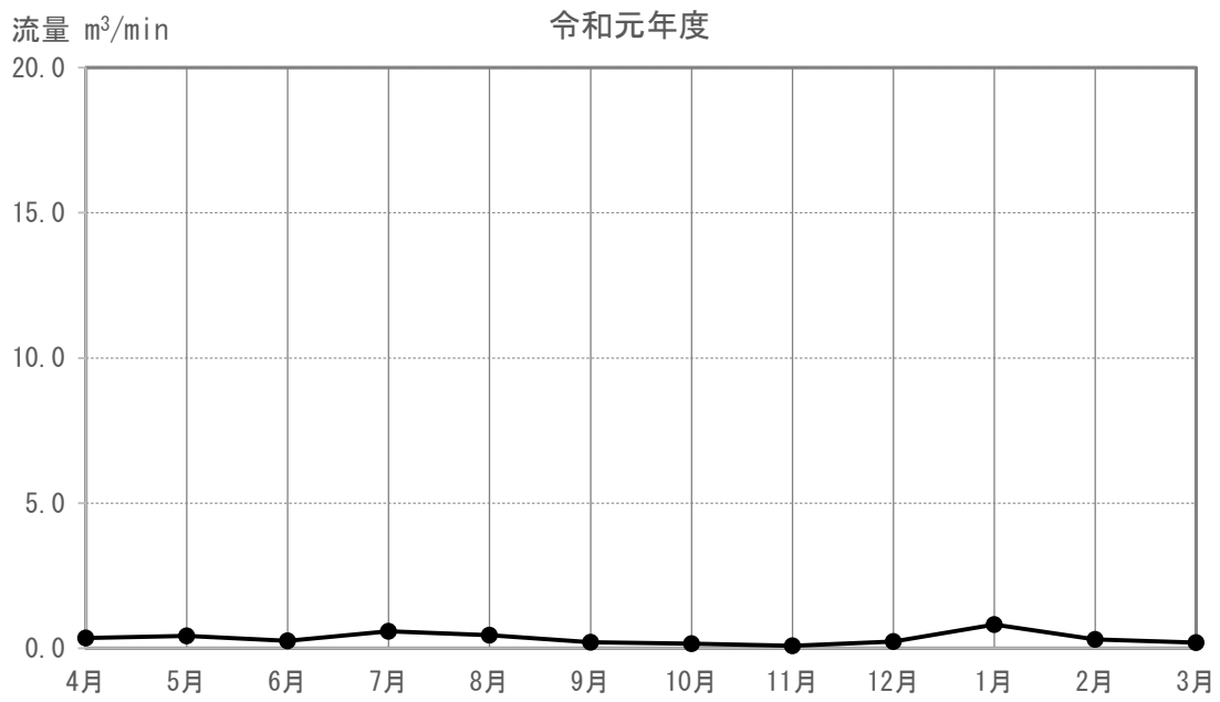
図 3-5-4-2 (43) 河川の流量の調査結果 (E-127)
