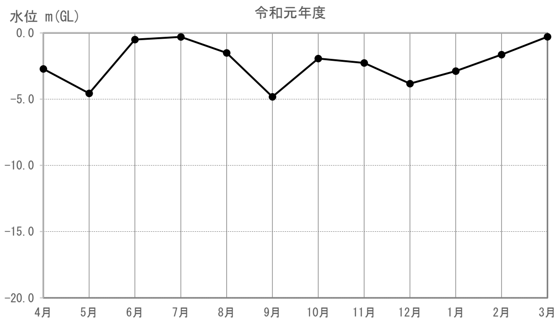
図 3-5-4-1(46) 地下水の水位（又は水量）の調査結果(M-104)
