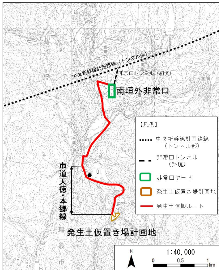
図 3-8-2-1 (2) 調査地点 (騒音)
