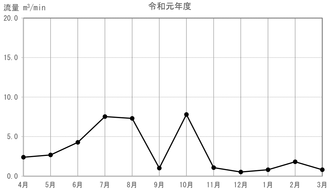
図 3-5-4-2(133) 河川の流量の調査結果(T-121)
