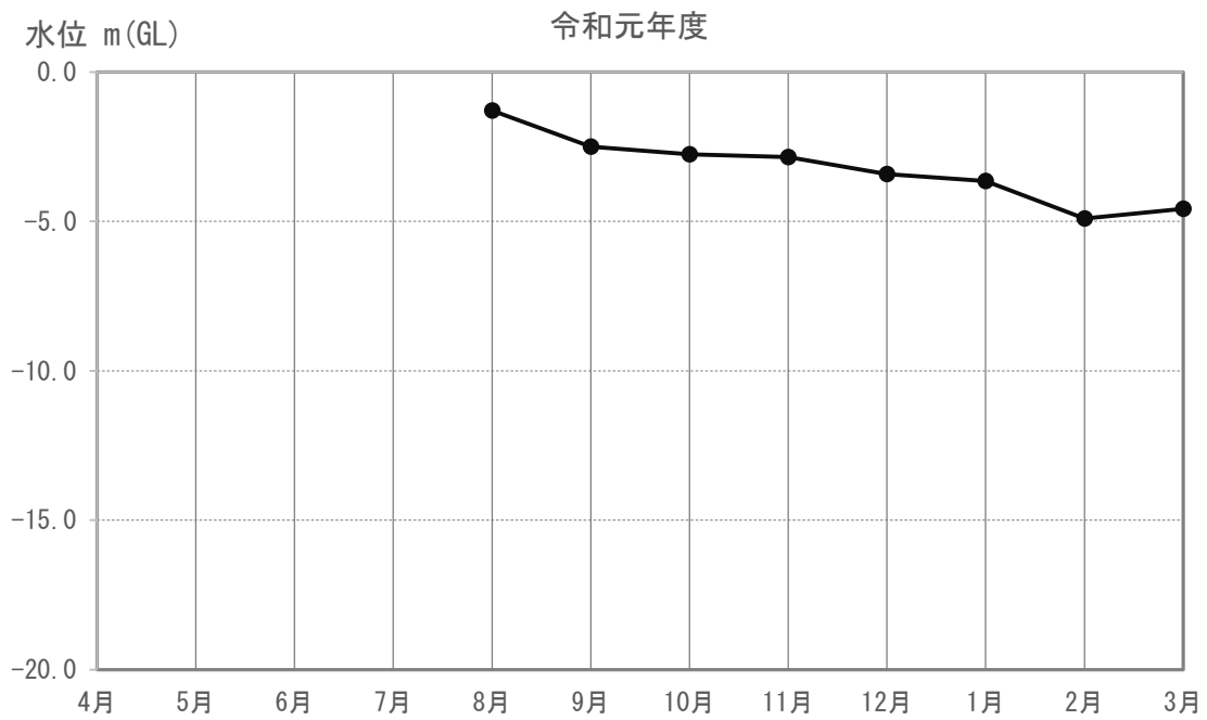
図 3-5-4-1 (25) 地下水の水位（又は水量）の調査結果 (N-138)
