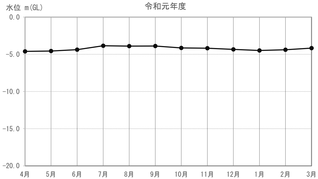
図 3-5-4-1(35) 地下水の水位（又は水量）の調査結果(E-106)
