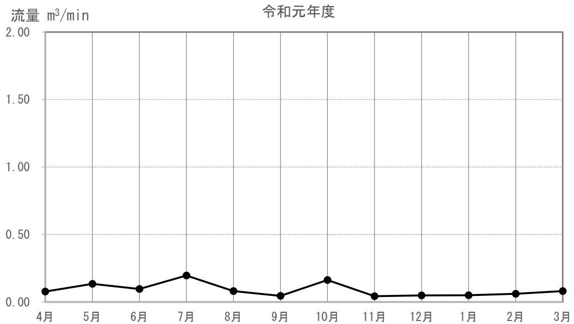
図 3-5-4-2(88) 河川の流量の調査結果(M-145)
