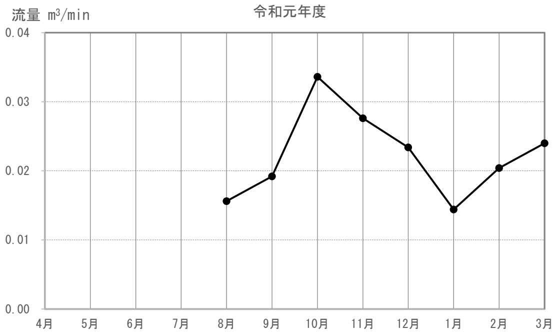
図 3-5-4-2(27) 河川の流量の調査結果 (N-156)
