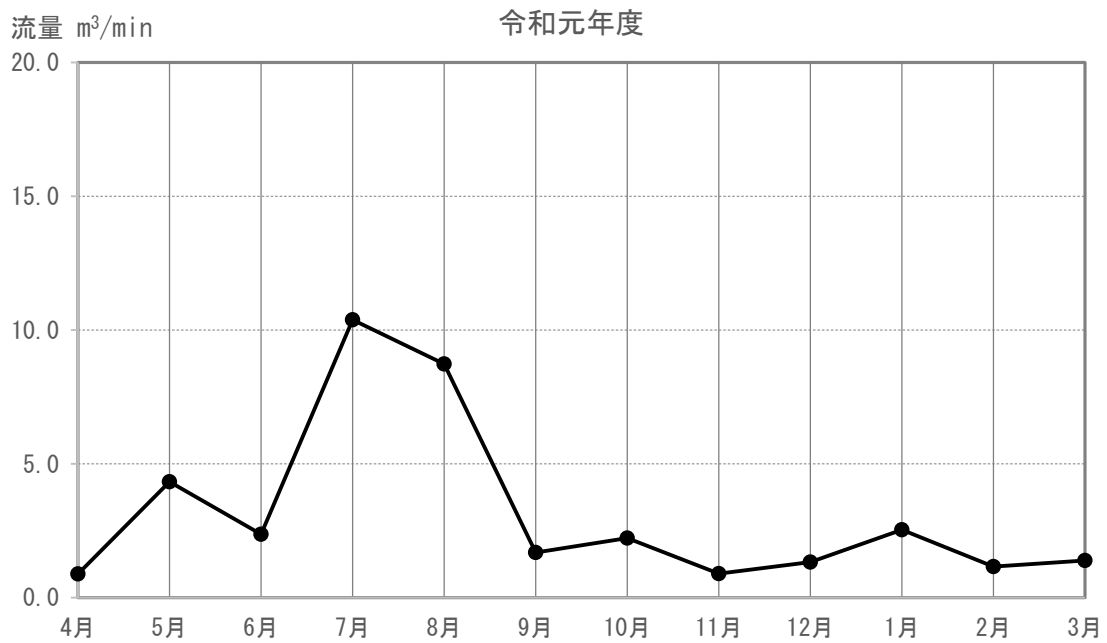
図 3-5-4-2(110) 河川の流量の調査結果 (K-116)
