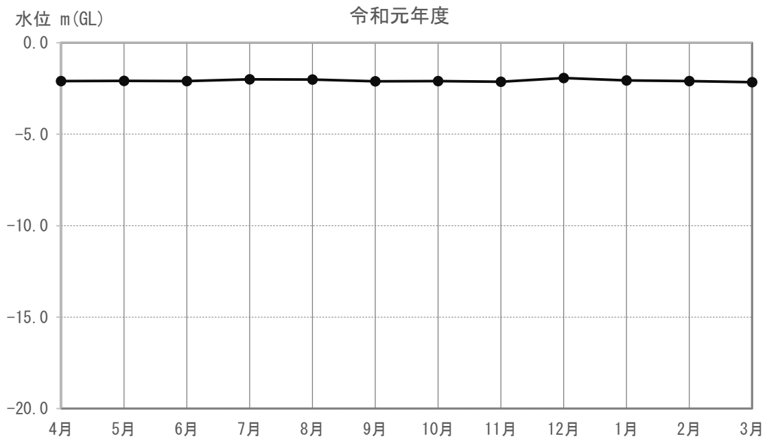
図 3-5-4-1 (61) 地下水の水位（又は水量）の調査結果 (K-105)
