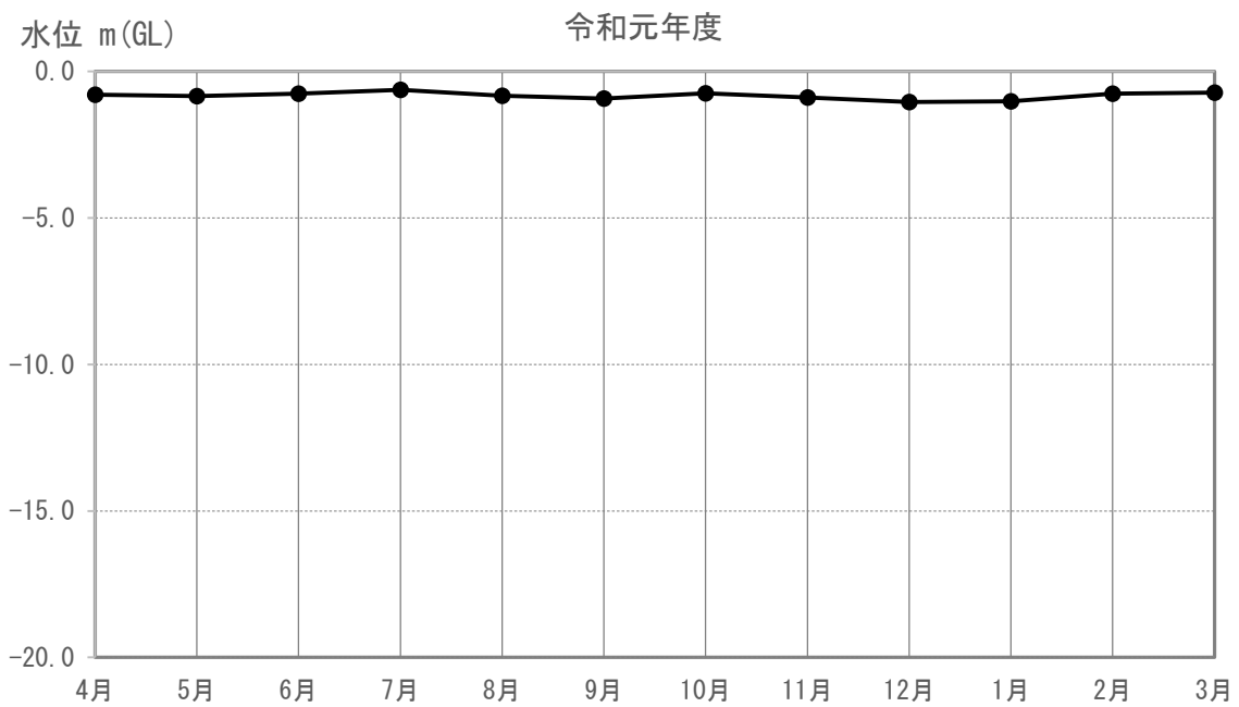
図 3-5-4-1 (56) 地下水の水位（又は水量）の調査結果 (M-114)
