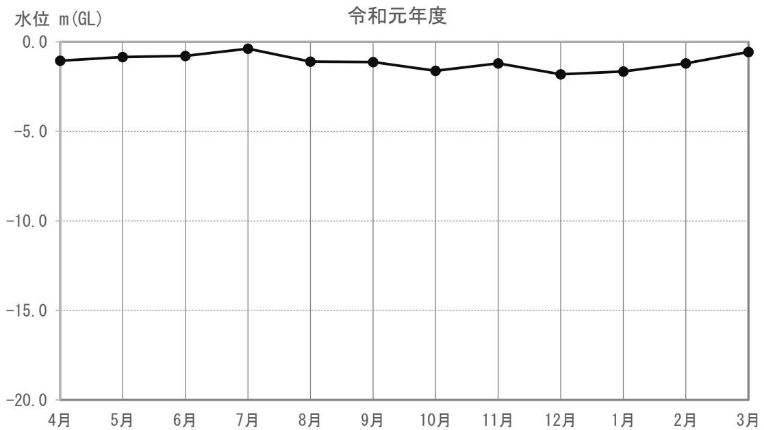
図 3-5-4-1(36) 地下水の水位（又は水量）の調査結果(E-107)
