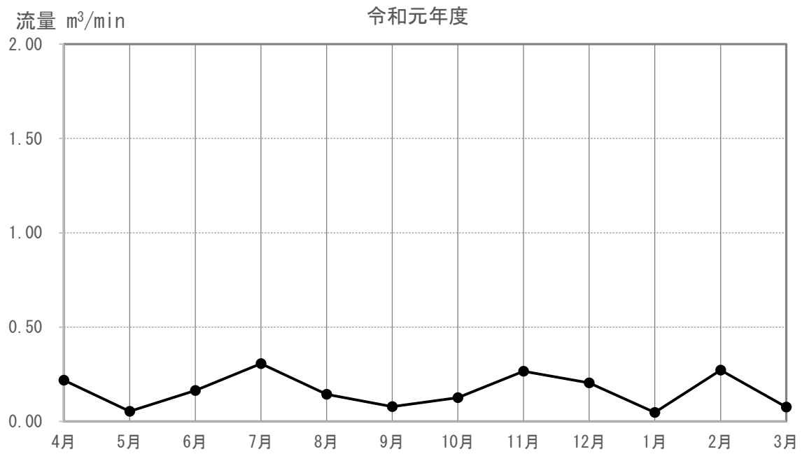
図 3-5-4-2(93) 河川の流量の調査結果(M-150)
