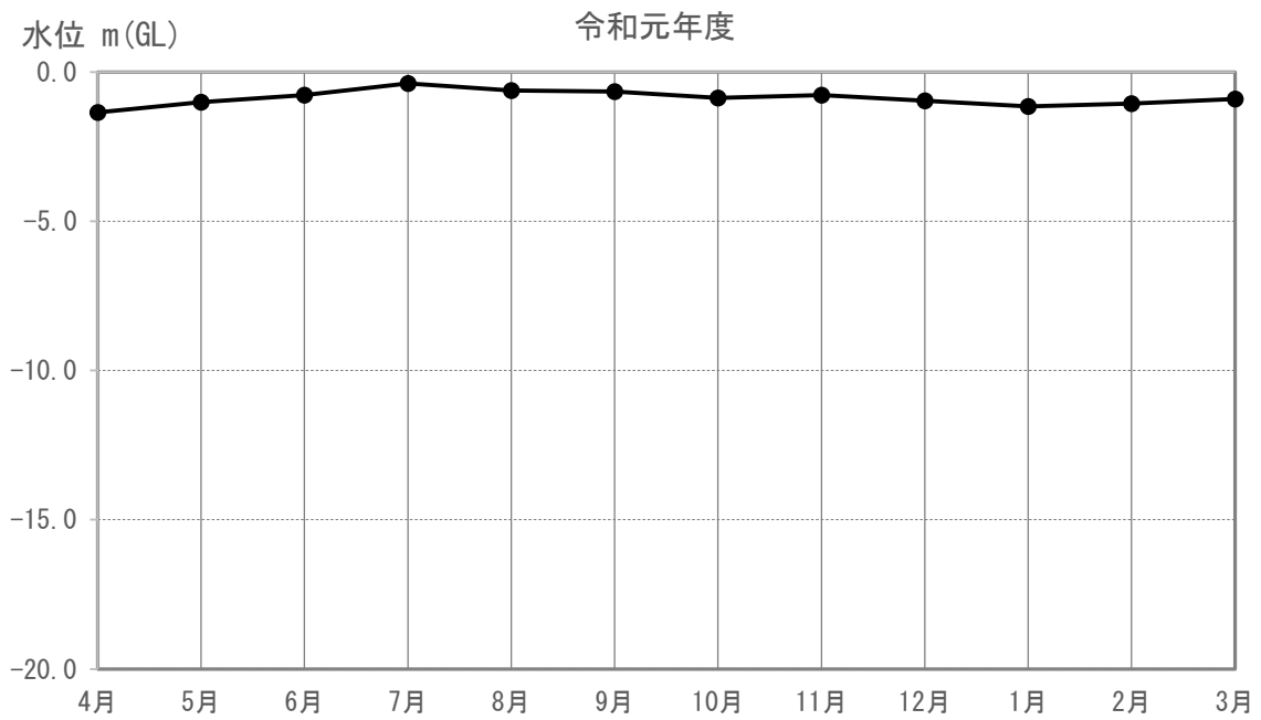
図 3-5-4-1(48) 地下水の水位（又は水量）の調査結果(M-106)
