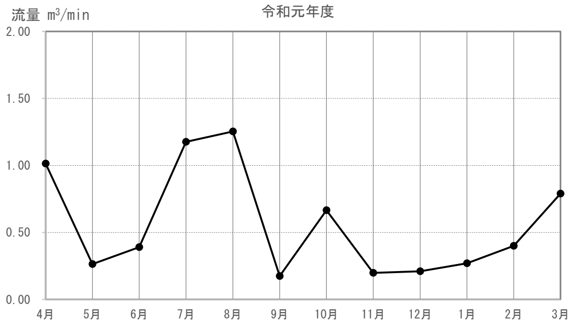
図 3-5-4-2(70) 河川の流量の調査結果(M-127)
