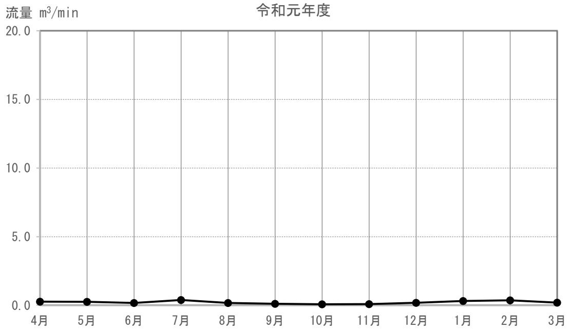
図 3-5-4-2(103) 河川の流量の調査結果(K-109)
