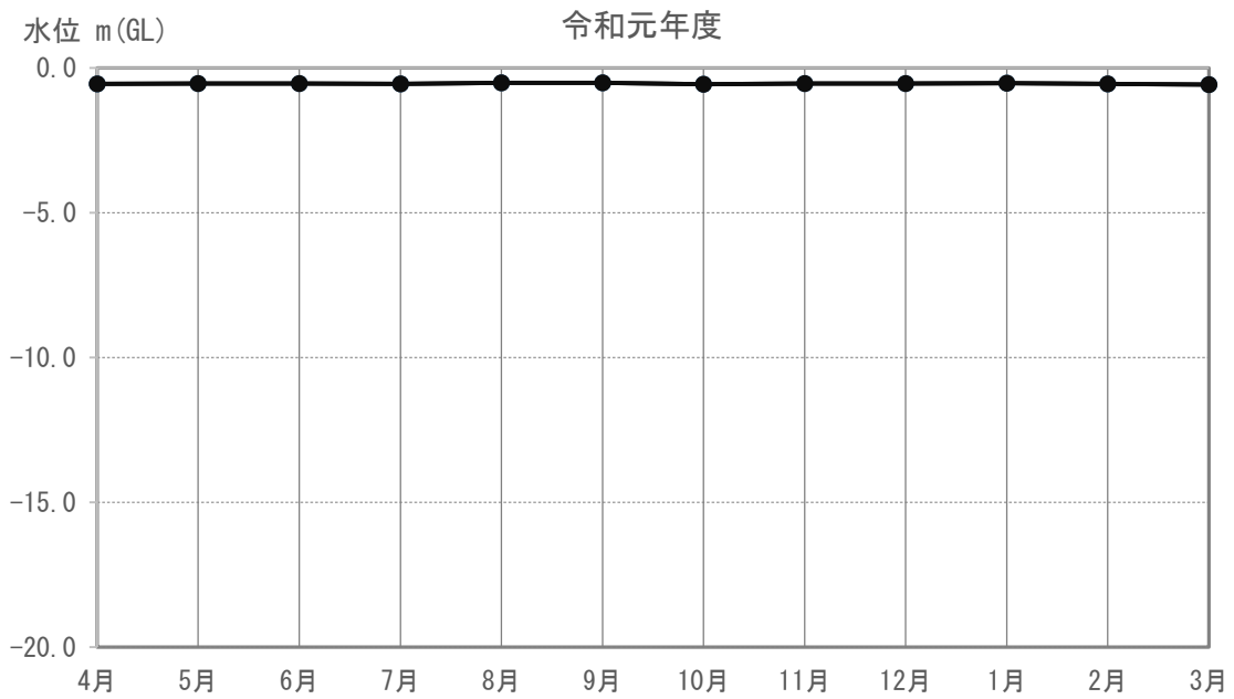
図 3-5-4-1 (30) 地下水の水位（又は水量）の調査結果 (E-101)
