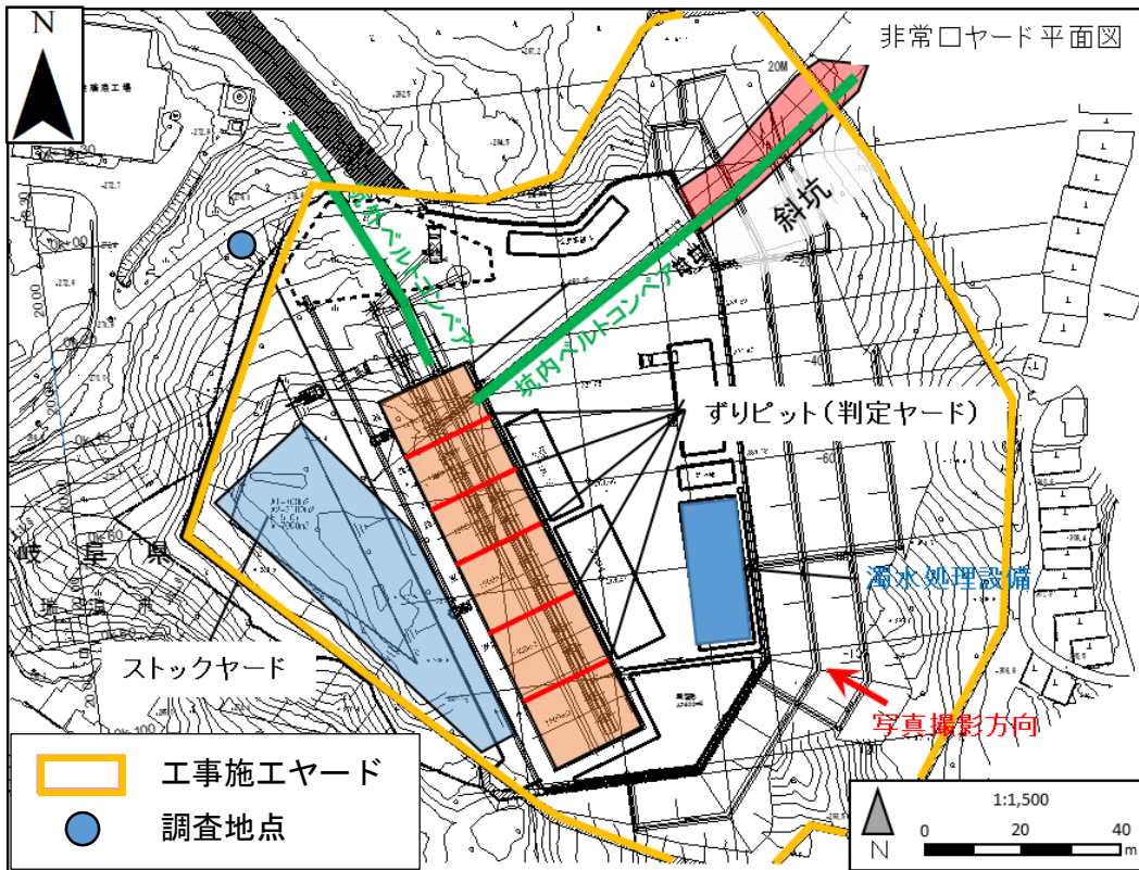
図 参-2(6) 常時計測の実施地点 (03 南垣外非常口)
