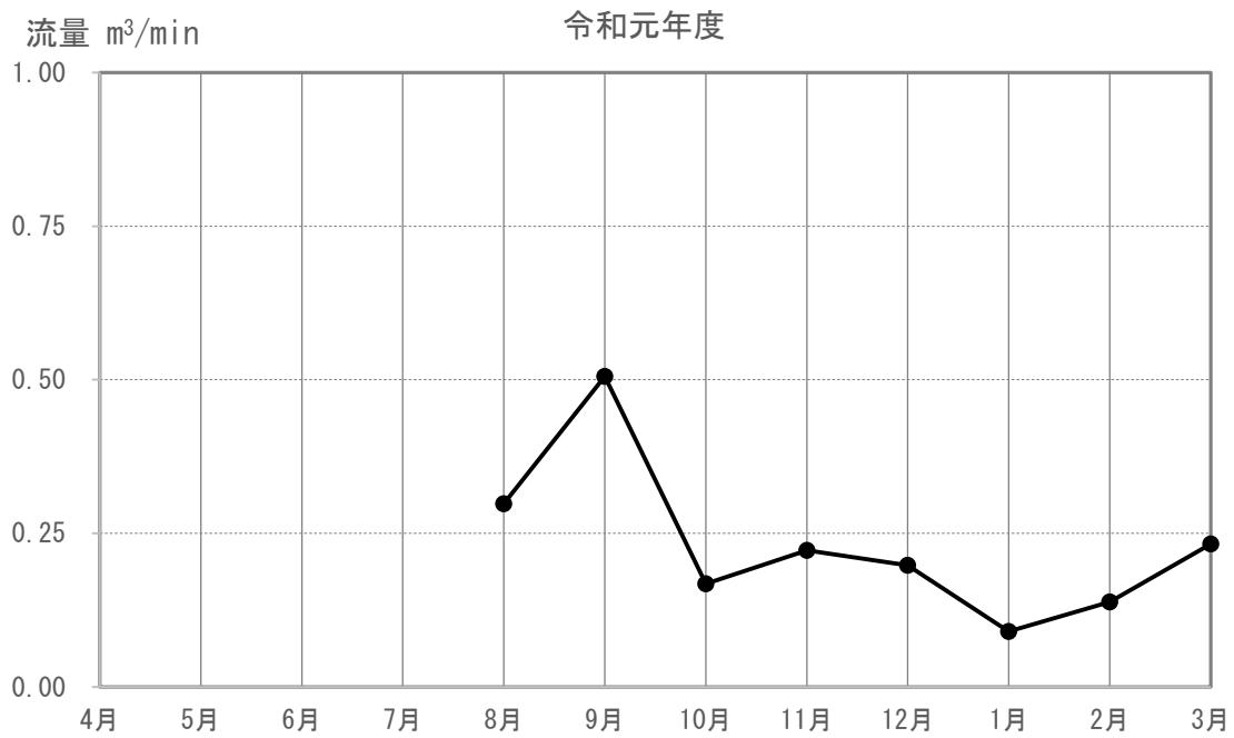
図 3-5-4-2(19) 河川の流量の調査結果 (N-148)
