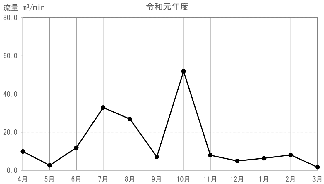
図 3-5-4-2(119) 河川の流量の調査結果(T-107)
