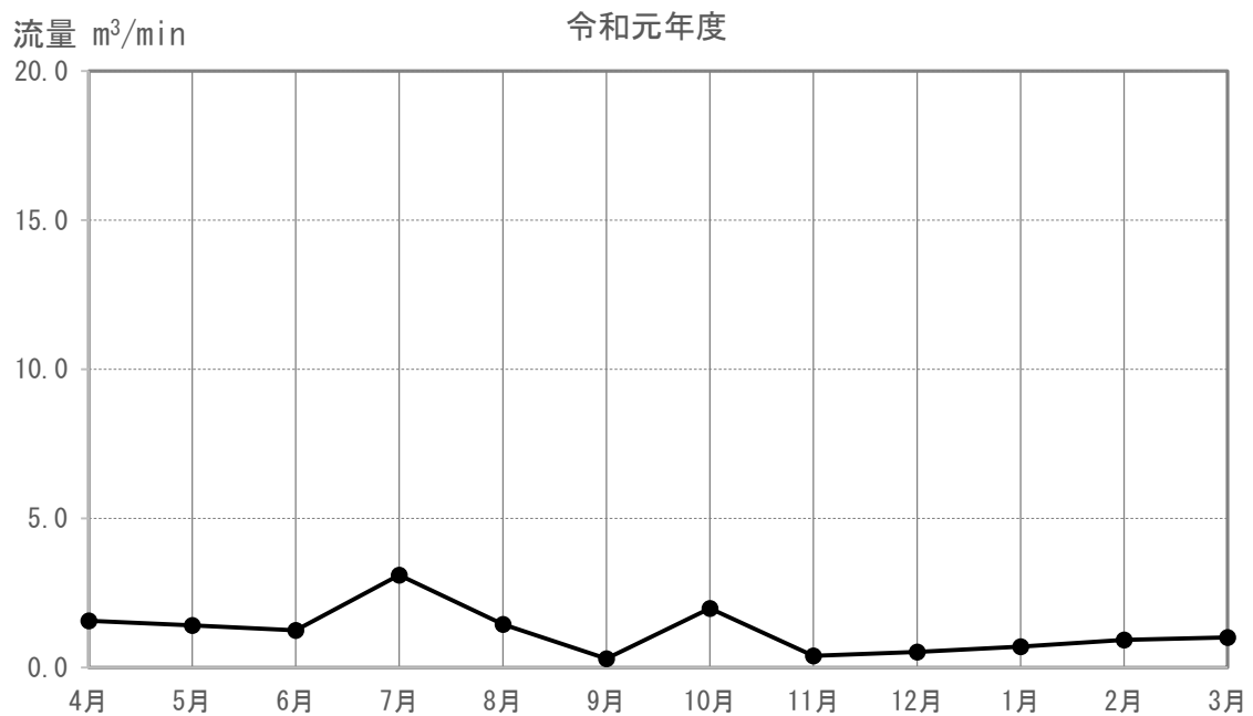
図 3-5-4-2(76) 河川の流量の調査結果(M-133)
