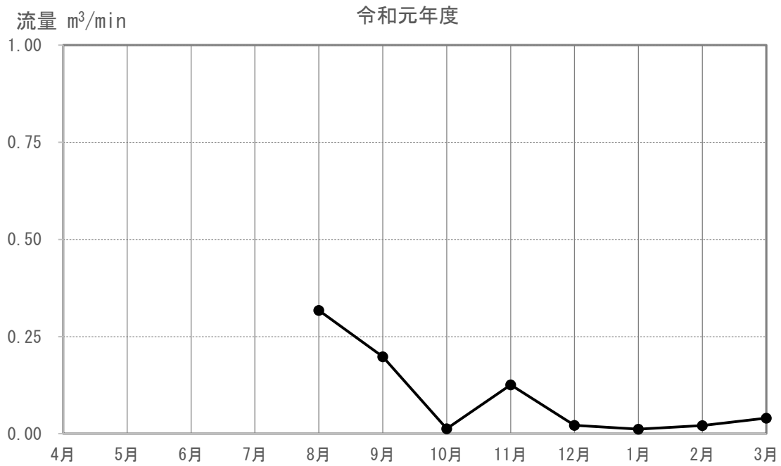
図 3-5-4-2(28) 河川の流量の調査結果 (N-157)
