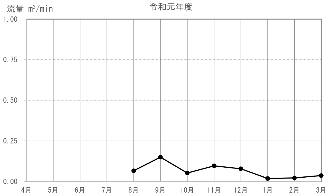
図 3-5-4-2 (25) 河川の流量の調査結果 (N-154)
