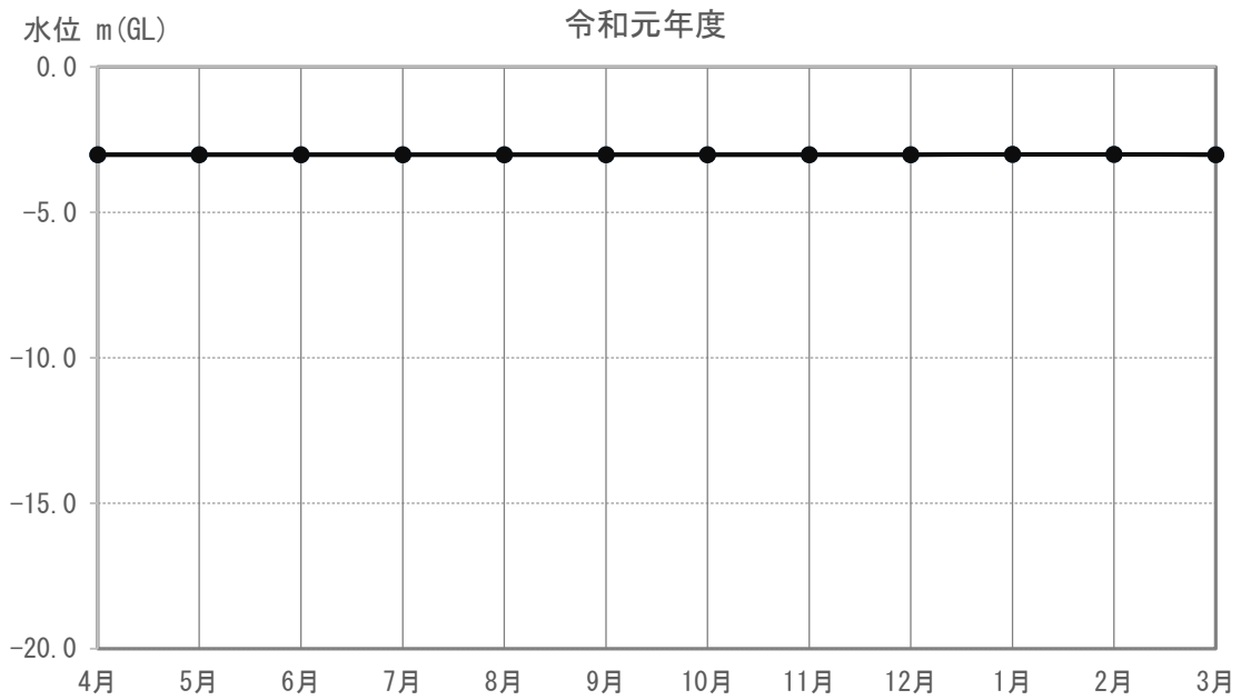
図 3-5-4-1(31) 地下水の水位（又は水量）の調査結果(E-102)
