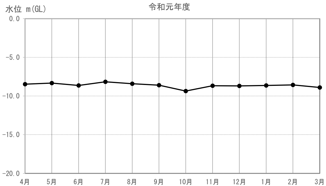
図 3-5-4-1(44) 地下水の水位（又は水量）の調査結果(M-102)
