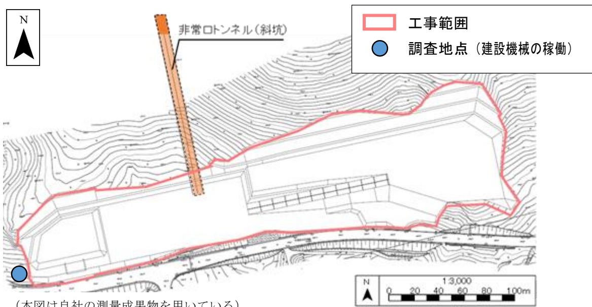
図 3-3-3-1(2) 工事最盛期のモニタリングの実施地点（振動）（02 瀬戸）
