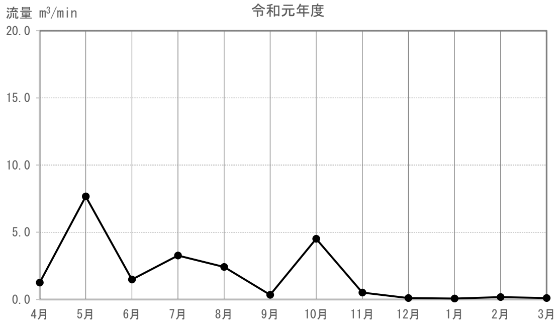
図 3-5-4-2(131) 河川の流量の調査結果(T-119)
