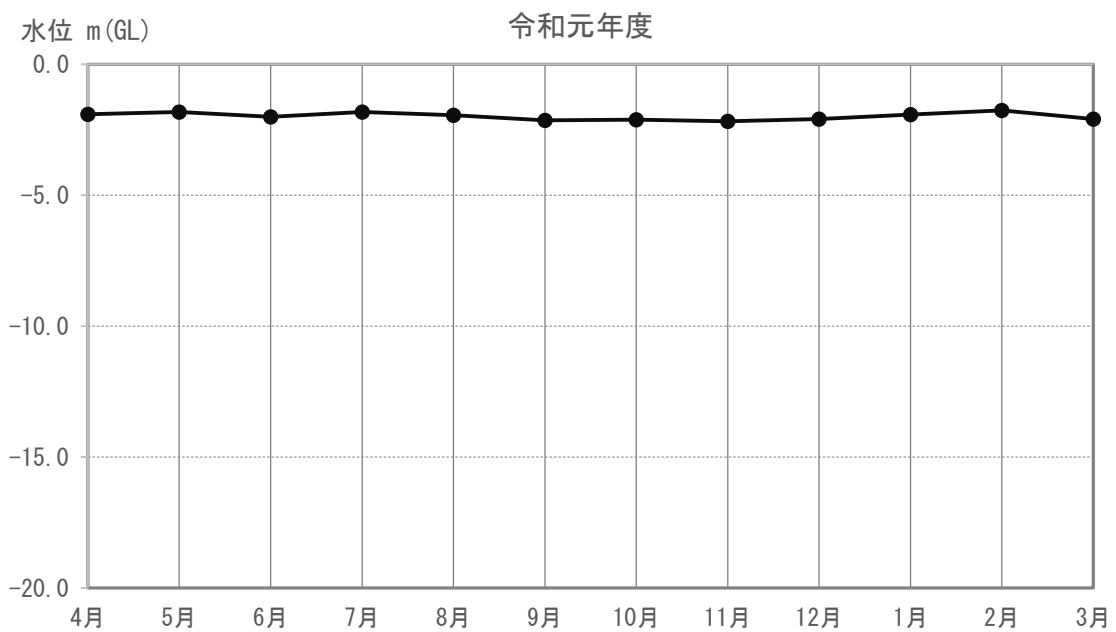
図 3-5-4-1(32) 地下水の水位（又は水量）の調査結果(E-103)
