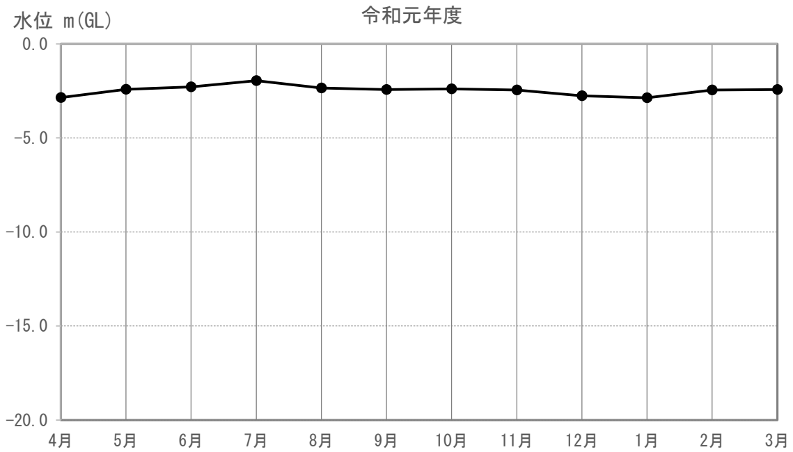
図 3-5-4-1(51) 地下水の水位（又は水量）の調査結果(M-109)
