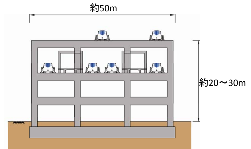
ホーム部の断面図
