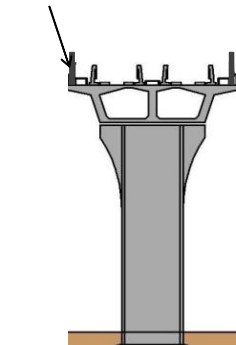
防音壁
