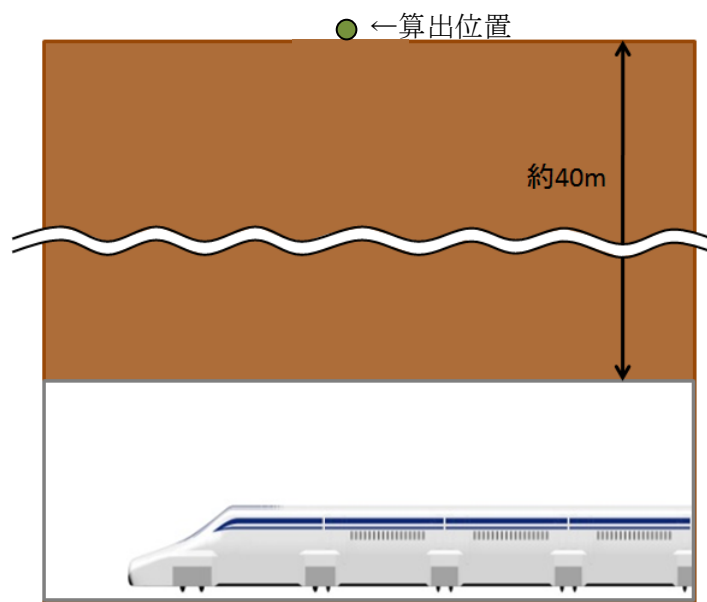
図 10-7-3-2 地上における磁界の算出位置イメージ（ケース 2）
