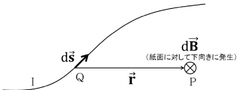
図 10-7-1-1 ビオ・サバルの法則概念図
