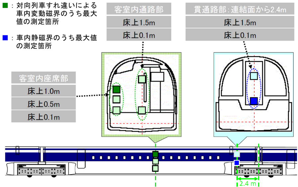
図 10-5-3 車内の磁界の測定箇所
