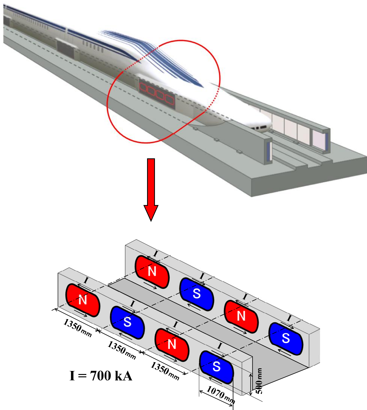
図 10-7-1-2 超電導磁石を拡大した概略図（磁界の算出にあたっての前提条件）
