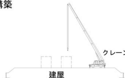
図 3-4-18 保守基地における施工概要
