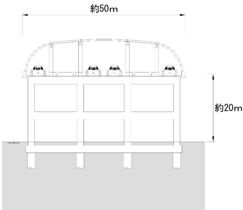
図 3-4-6 地上駅の概要
