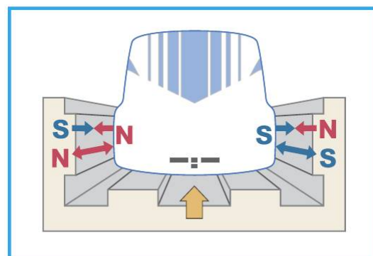
図 3-4-22 浮上の原理
