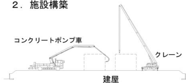
図 3-4-17 変電施設における施工概要
