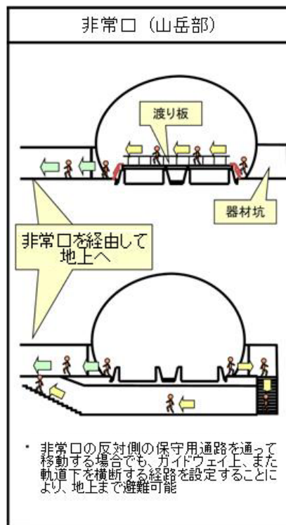
図 3-4-28 非常口における避難の概要
