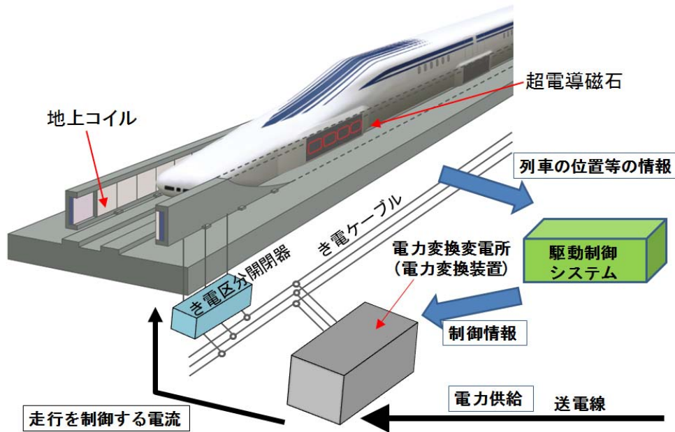
図 3-4-24 列車走行に関わる設備の概要
