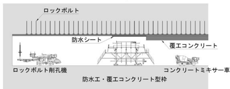
図 3-4-13 山岳トンネル部における施工概要
