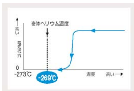
図 3-4-19 電気抵抗と温度の関係
