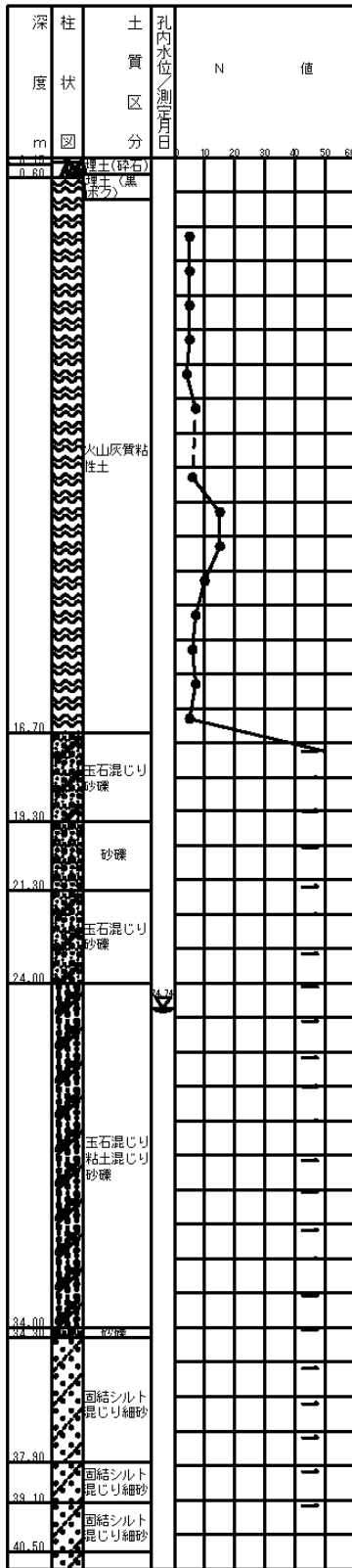
図 8-1-2(2) 地質柱状図 (地点番号 02)
