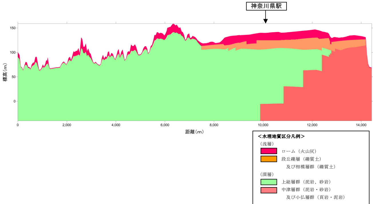
図 6-3-2-6 地下地質区分
