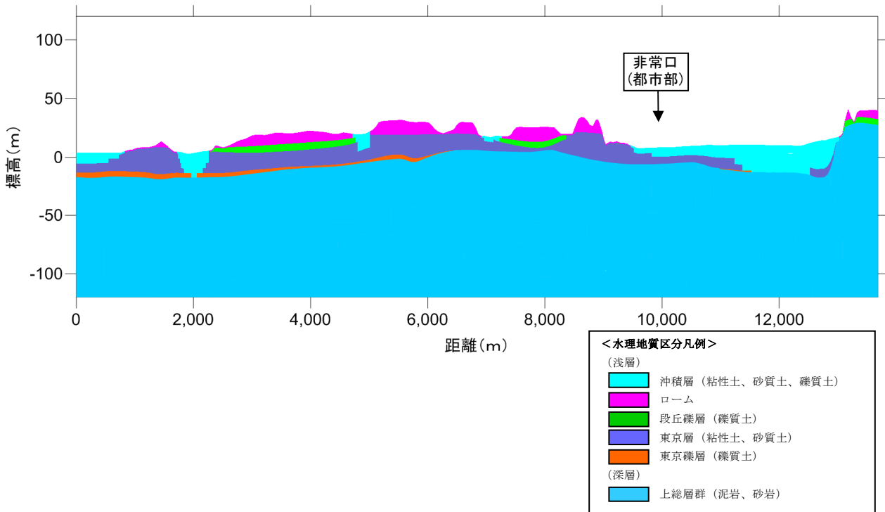
図 6-3-2-3 地下地質区分
