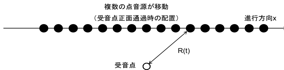
図 2-7-2 音源モデル
