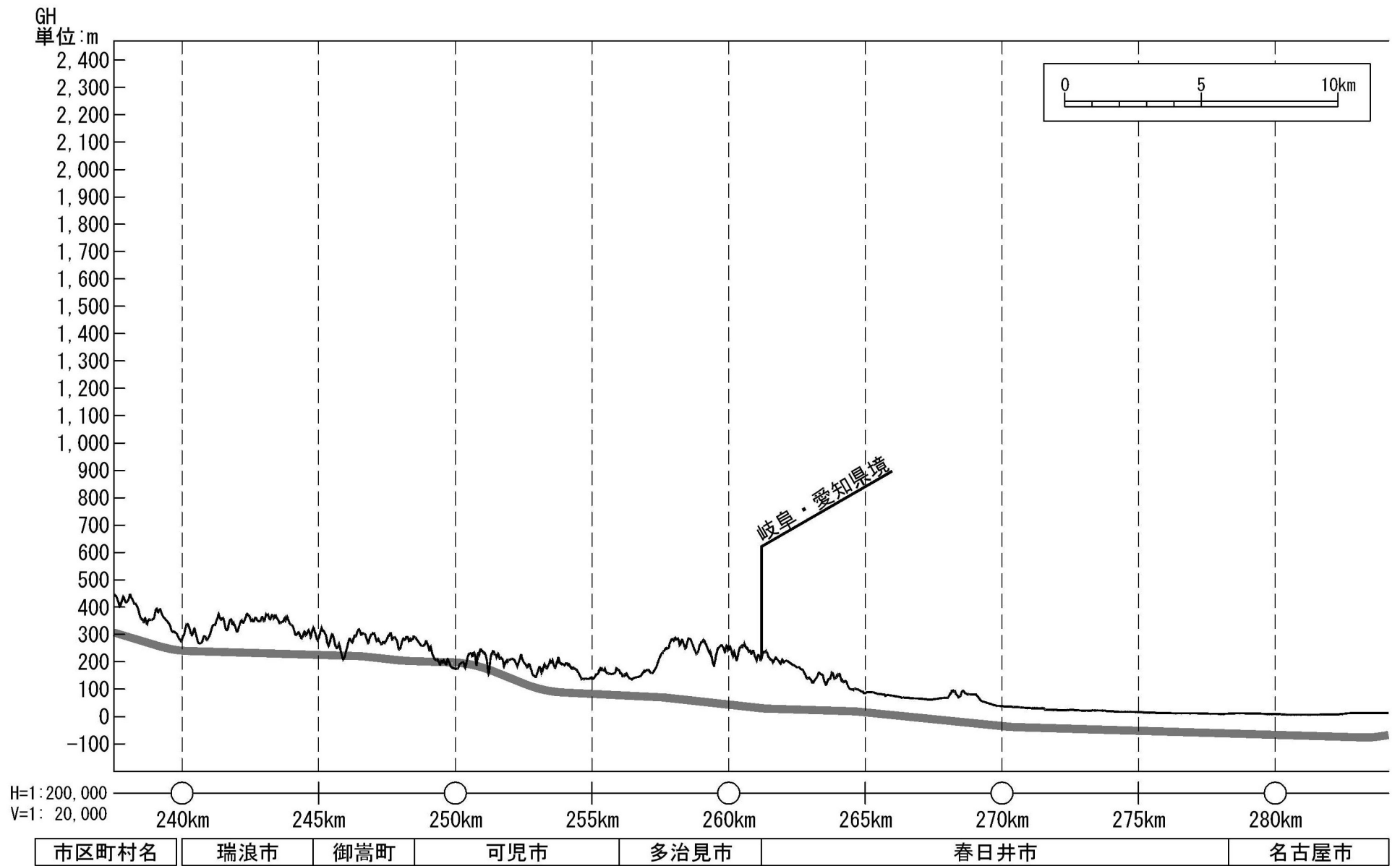
图 2-1(7) 路線概要 (縦断計画)
