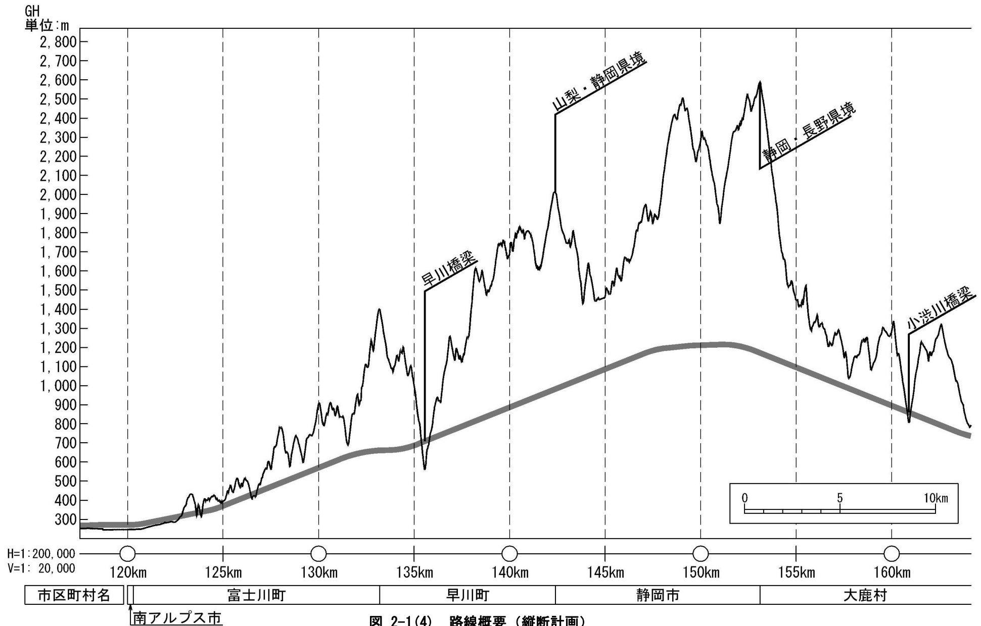
図 2-1(4) 路線概要 (縦断計画)
