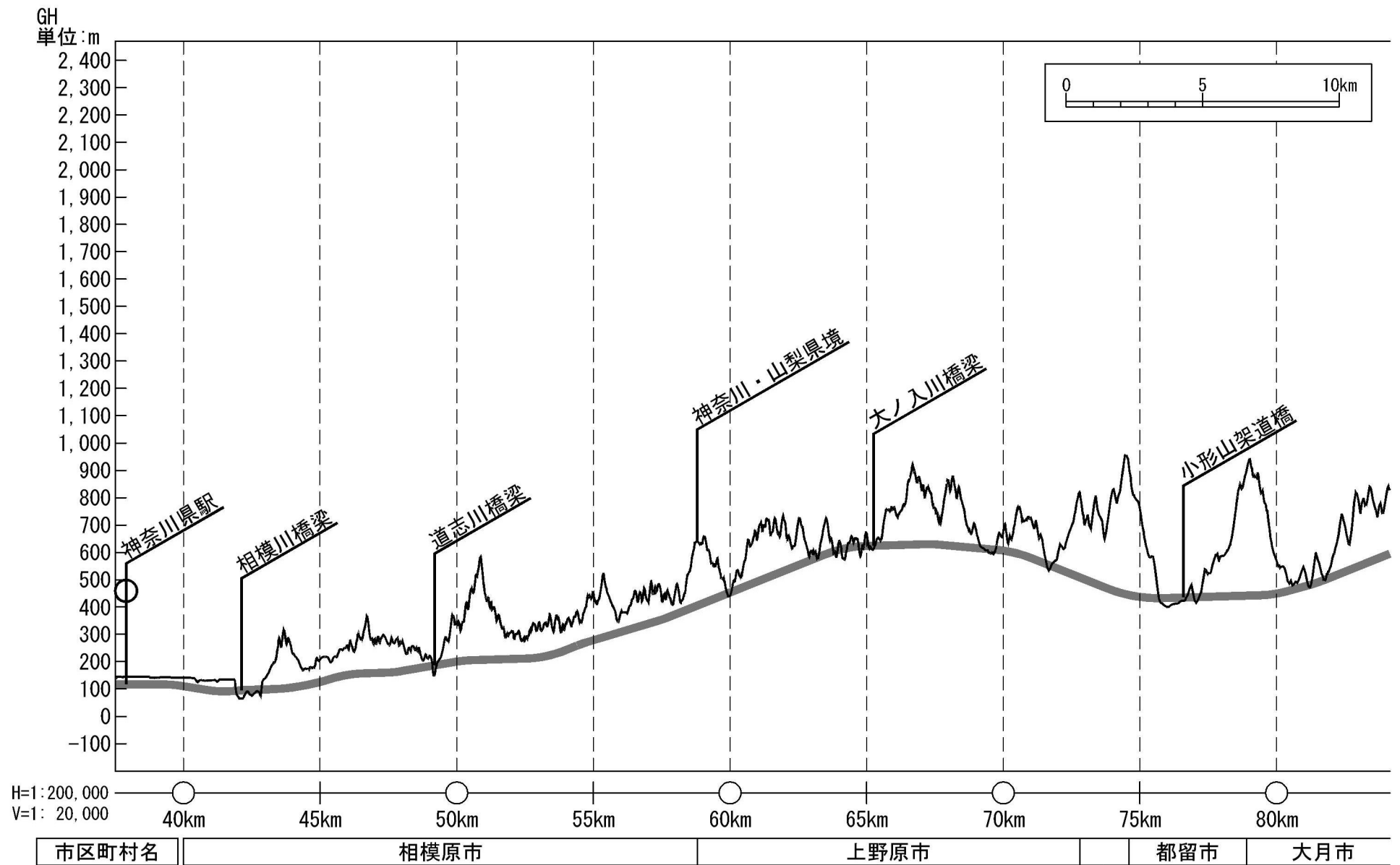
図 2-1(2) 路線概要(縦断計画)
