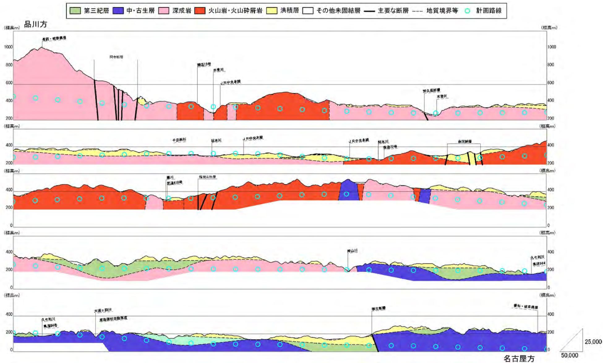
図 8-2-3-4 地質縦断図
