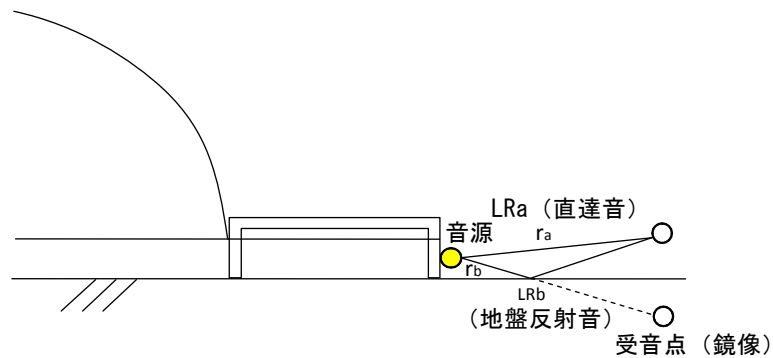
図 8-1-2-8 予測式の模式図
