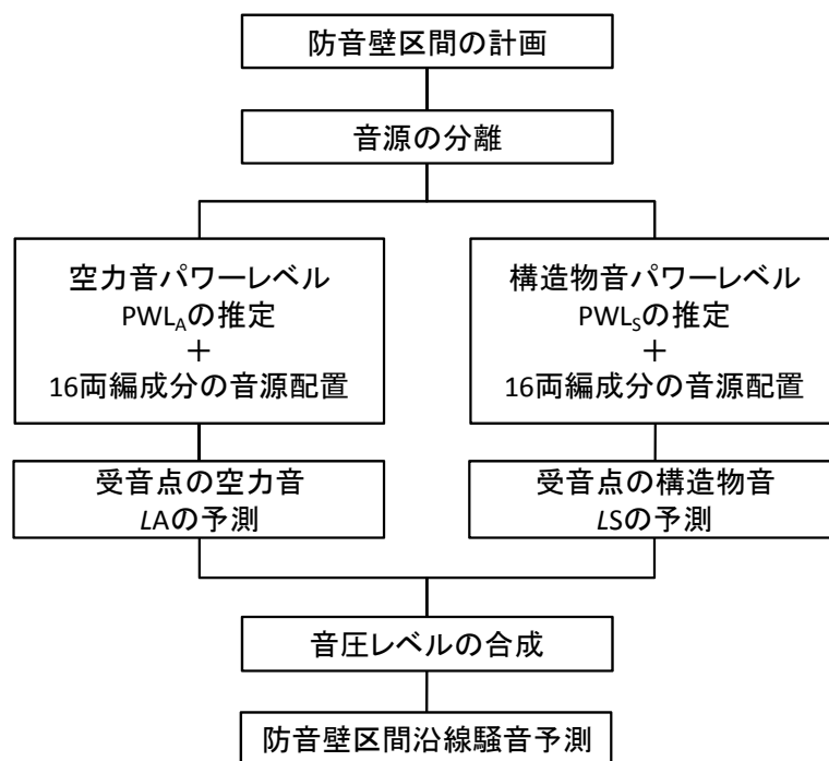
図 8-1-2-10 防音壁区間の騒音予測フロー
