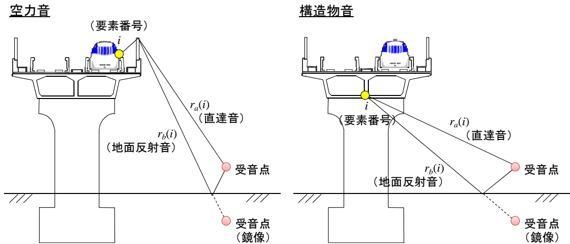
図 8-1-2-11 ある時刻における防音壁区間の予測式の模式図
