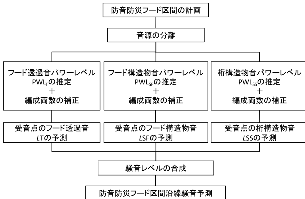
図 8-1-2-12 防音防災フード区間の騒音予測フロー
