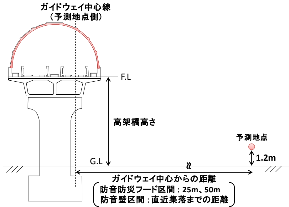
図 8-1-2-14(1) 予測地点模式図 (市町の代表地点)
