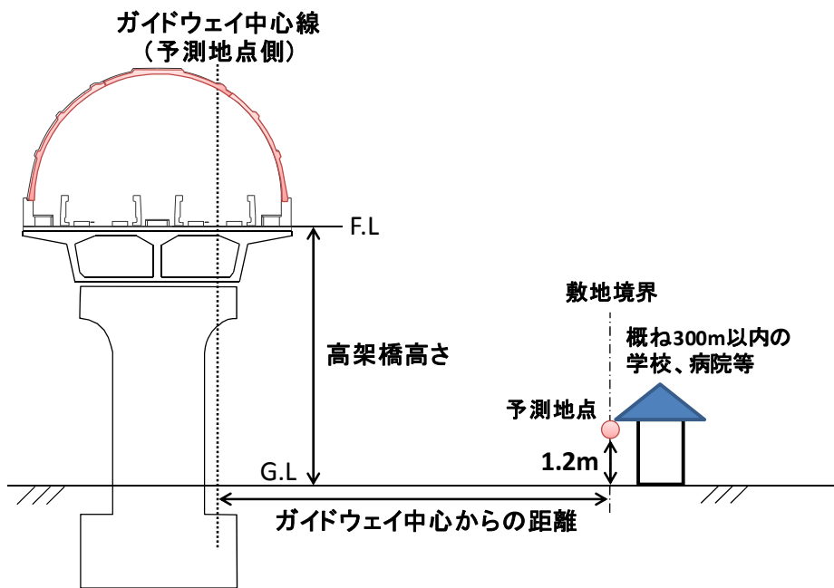
図 8-1-2-14(2) 予測地点模式図 (路線近傍の学校、病院等)
