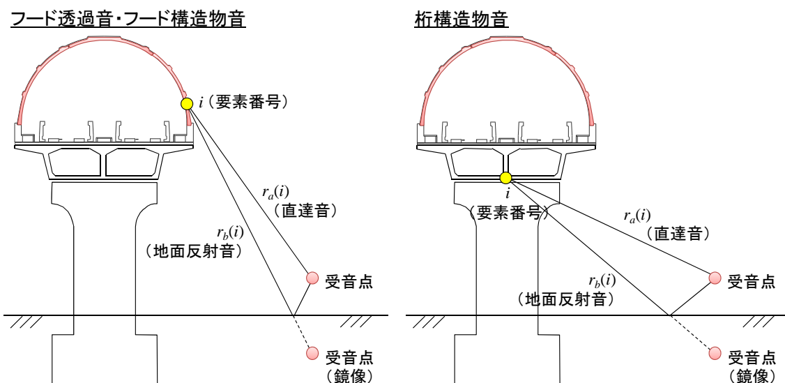
図 8-1-2-13 防音防災フード区間の予測式の模式図
