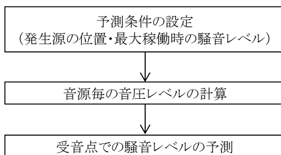
図 8-1-2-7 鉄道施設（換気施設）の供用における騒音予測フロー
