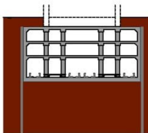
図 3-4-22 駅部における施工イメージ
