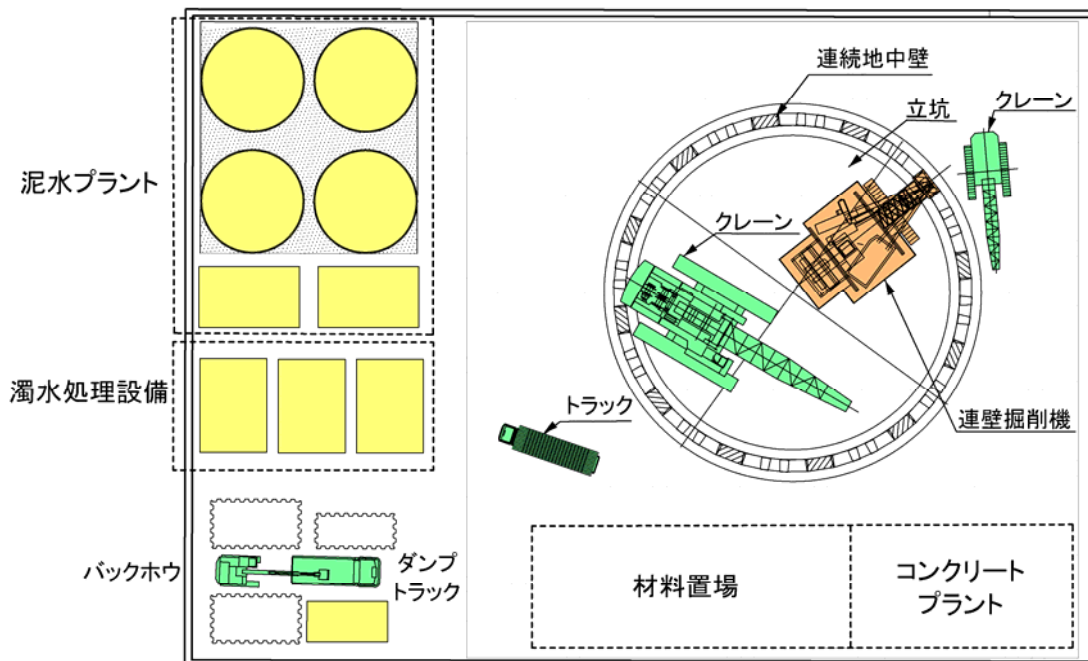
図 3-4-26 (1) 立坑の施工ヤードのイメージ (立坑構築時)
