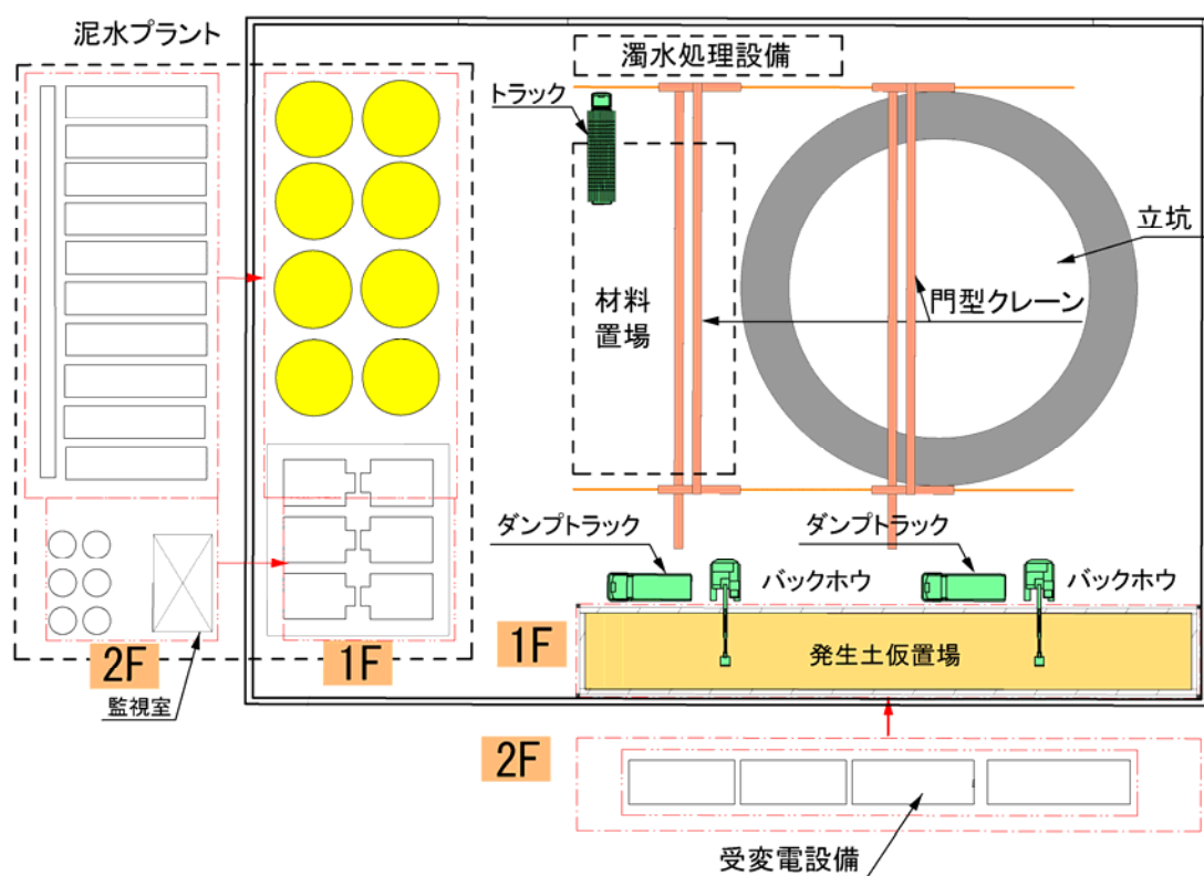
図 3-4-26 (2) 立坑の施工ヤードのイメージ (シールド構築時)
