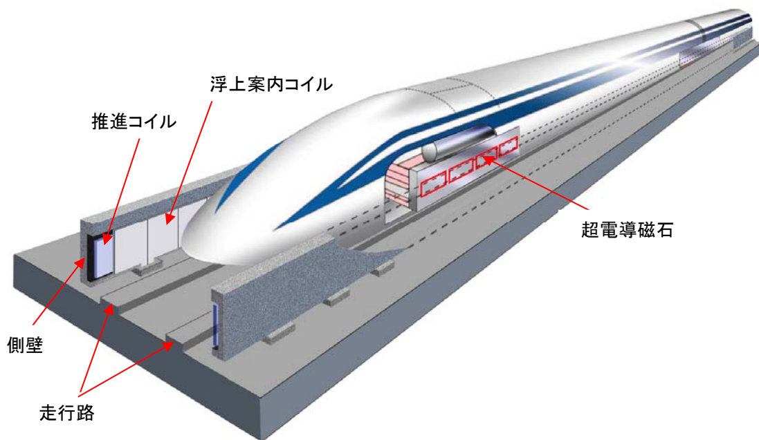
図 3-4-4 ガイドウェイの構成
