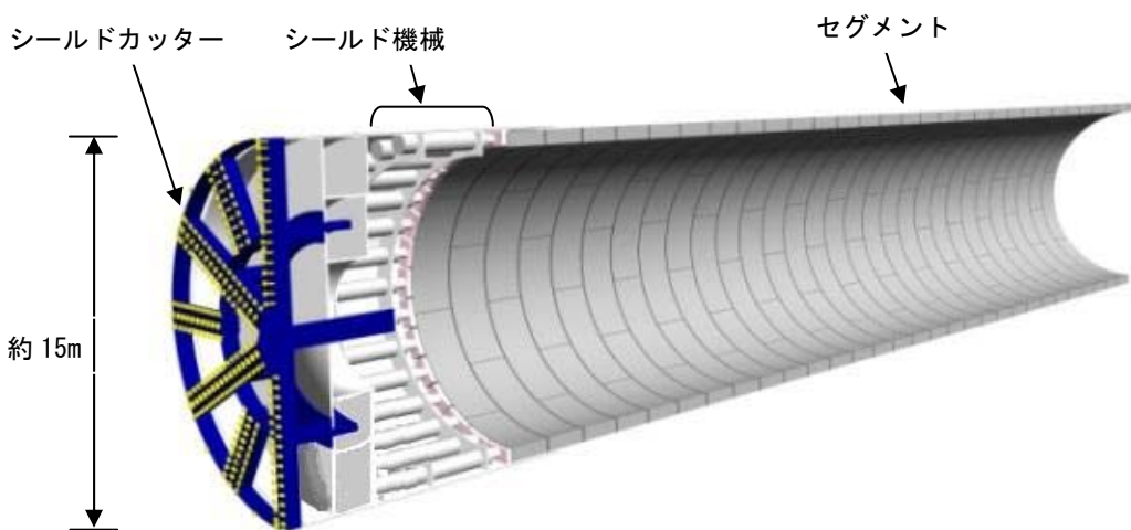
図 3-4-24 シールド機械（断面図）
