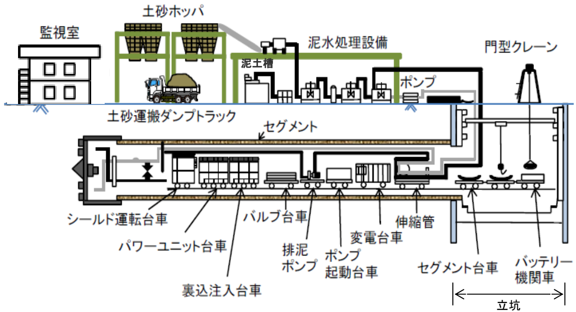
図 3-4-23 大深度地下トンネル部における施工イメージ（泥水式シールドの場合）
