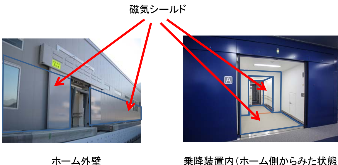
図 13-1-3-2 ホームへの磁気シールド設置の概念図
