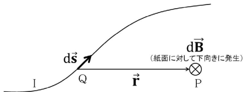
図 13-7-1-1 ビオ・サバルの法則概念図
