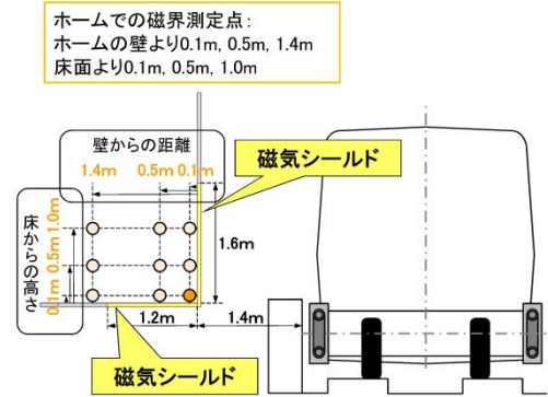
図 13-1-3-7 ホーム上の磁界の測定箇所
