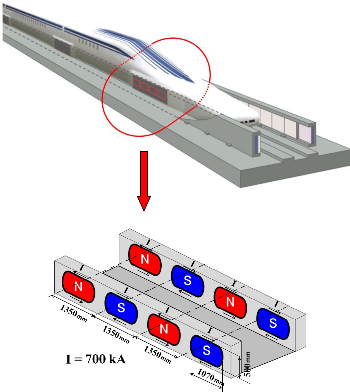
図 13-7-1-2 超電導磁石を拡大した概略図（磁界の算出にあたっての前提条件）
