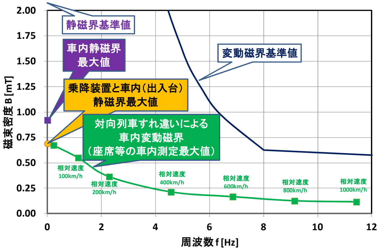
図 13-1-3-5 車内及び乗降装置と車内(出入台)の磁界の測定結果
