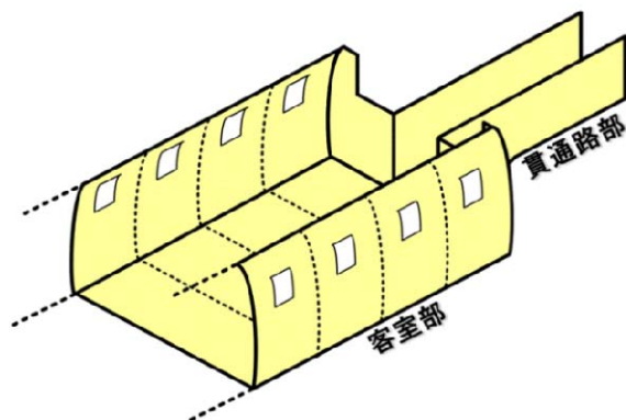
図 13-1-3-1 車内への磁気シールド設置の概念図
