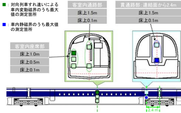
図 13-1-3-6 車内の磁界の測定箇所
