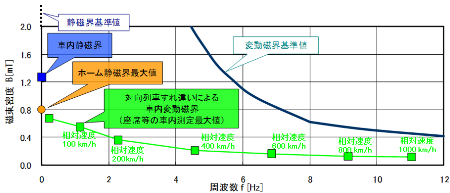
図 13-1-3-8 車内及びホームの磁界の測定結果
