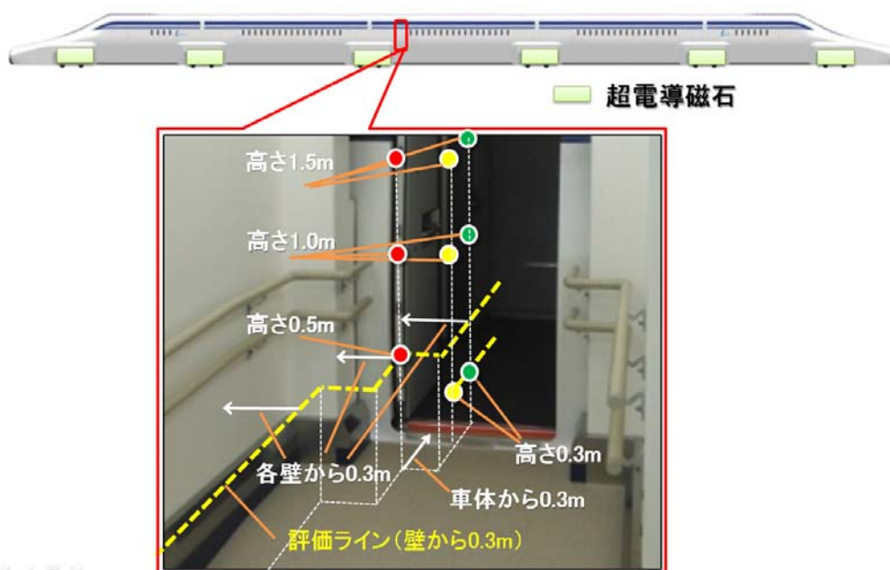
図 13-1-3-4 乗降装置と車内(出入台)の磁界の測定箇所
