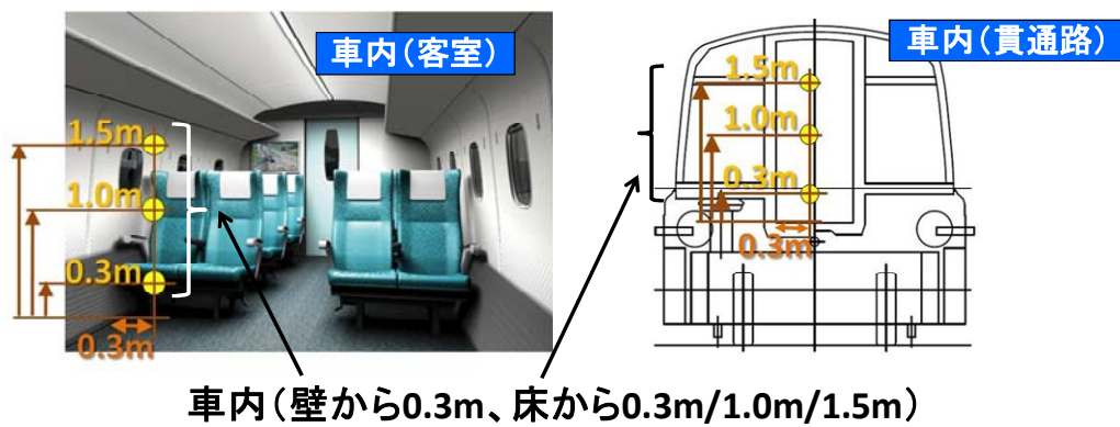
図 13-1-3-3 車内の磁界の測定箇所
