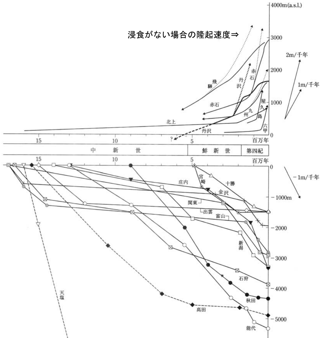
出典：日本の地形1 総説, 米倉ほか, 東京大学出版会, 2005 p. 308 (一部加筆) ※山脈の隆起については前期更新世・鮮新世テフラを指標とし、平野/盆地の沈下は深層試すいデータから算出
