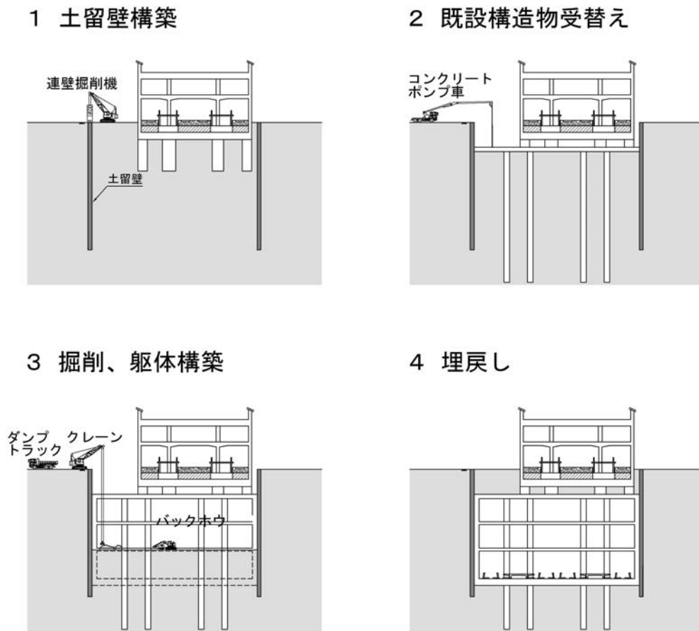
図 3-4-11 駅部における施工概要
