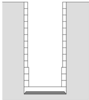
図 3-4-17 非常口の施工概要 (ケーソン工法の場合)
