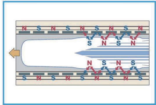
図 3-4-25 推進の原理
