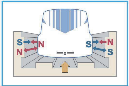
図 3-4-26 浮上の原理
