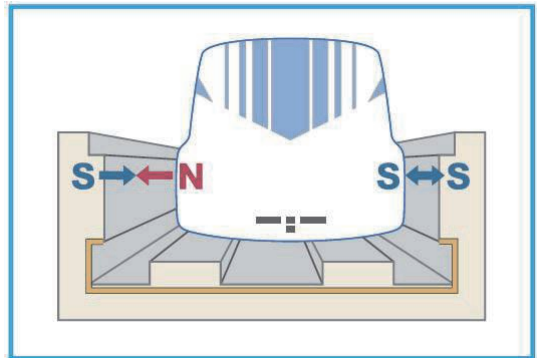
図 3-4-27 案内の原理
