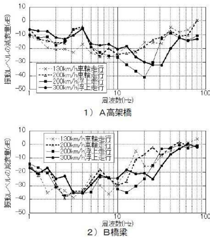
図-13 桁スラブ面から桁裏面にかけての1/3オクターブバンド振動レベルの減衰量
