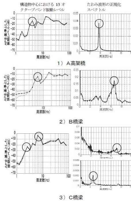
図-19 500km/h走行時の構造物中心における1/3オクターブバンド振動レベルと桁たわみの関係
