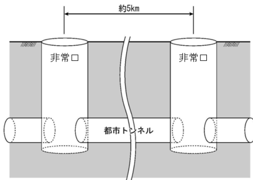
図 3-4-6-5 都市部の非常口の概要
