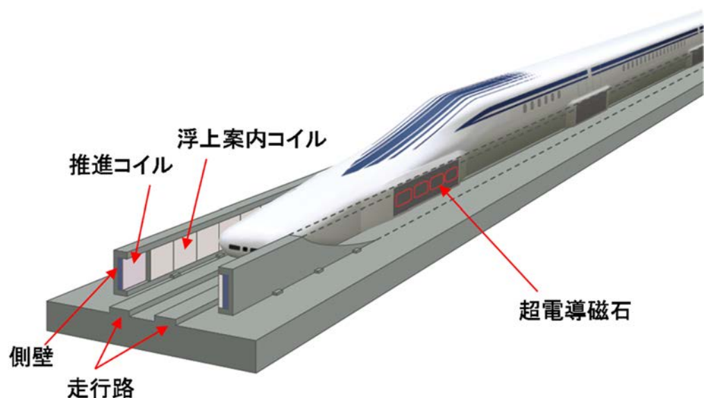
図 3-4-10-2 車両とガイドウェイの構成
