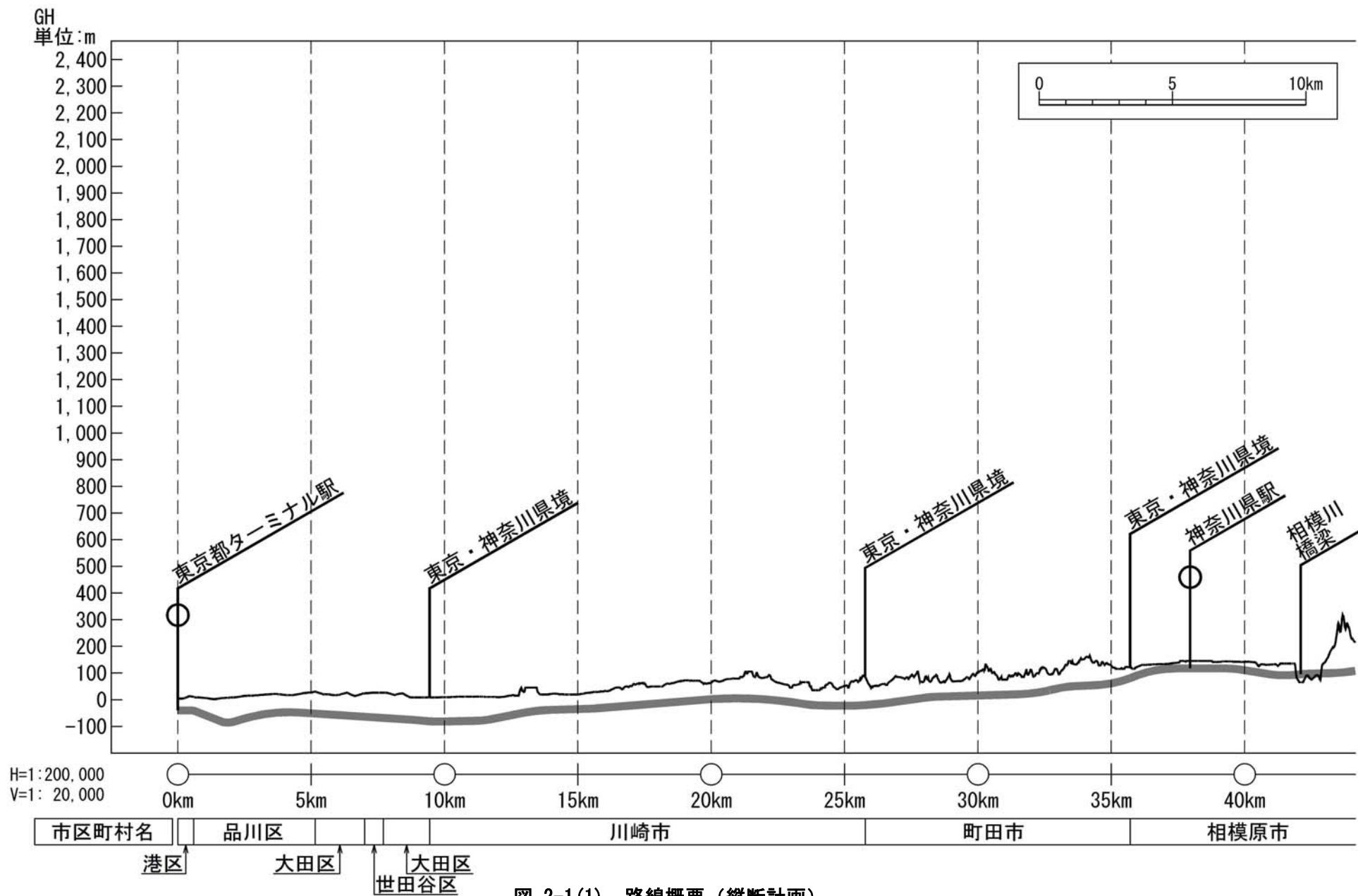
図 2-1(1) 路線概要 (縦断計画)
