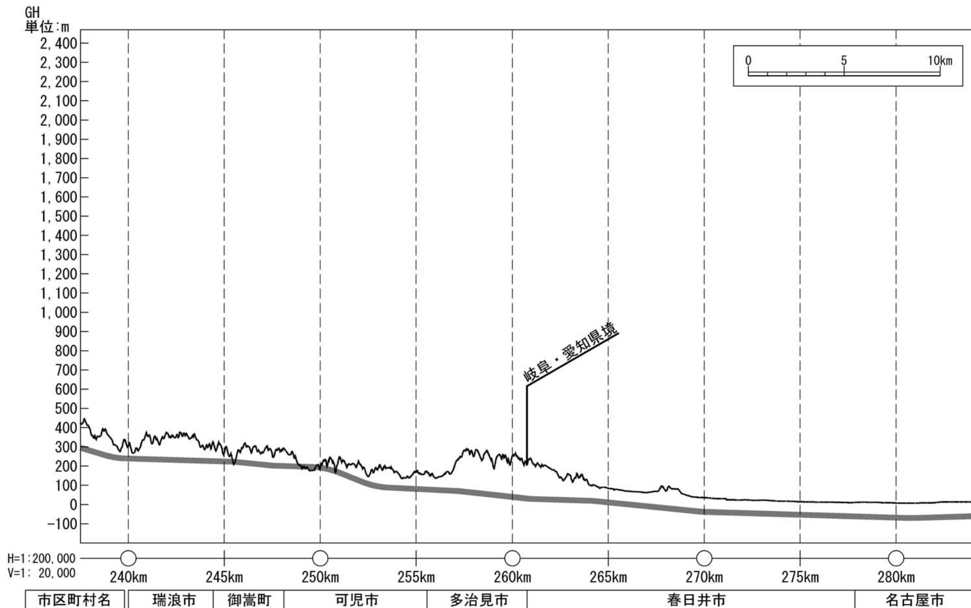
図 2-1(7) 路線概要 (縦断計画)
