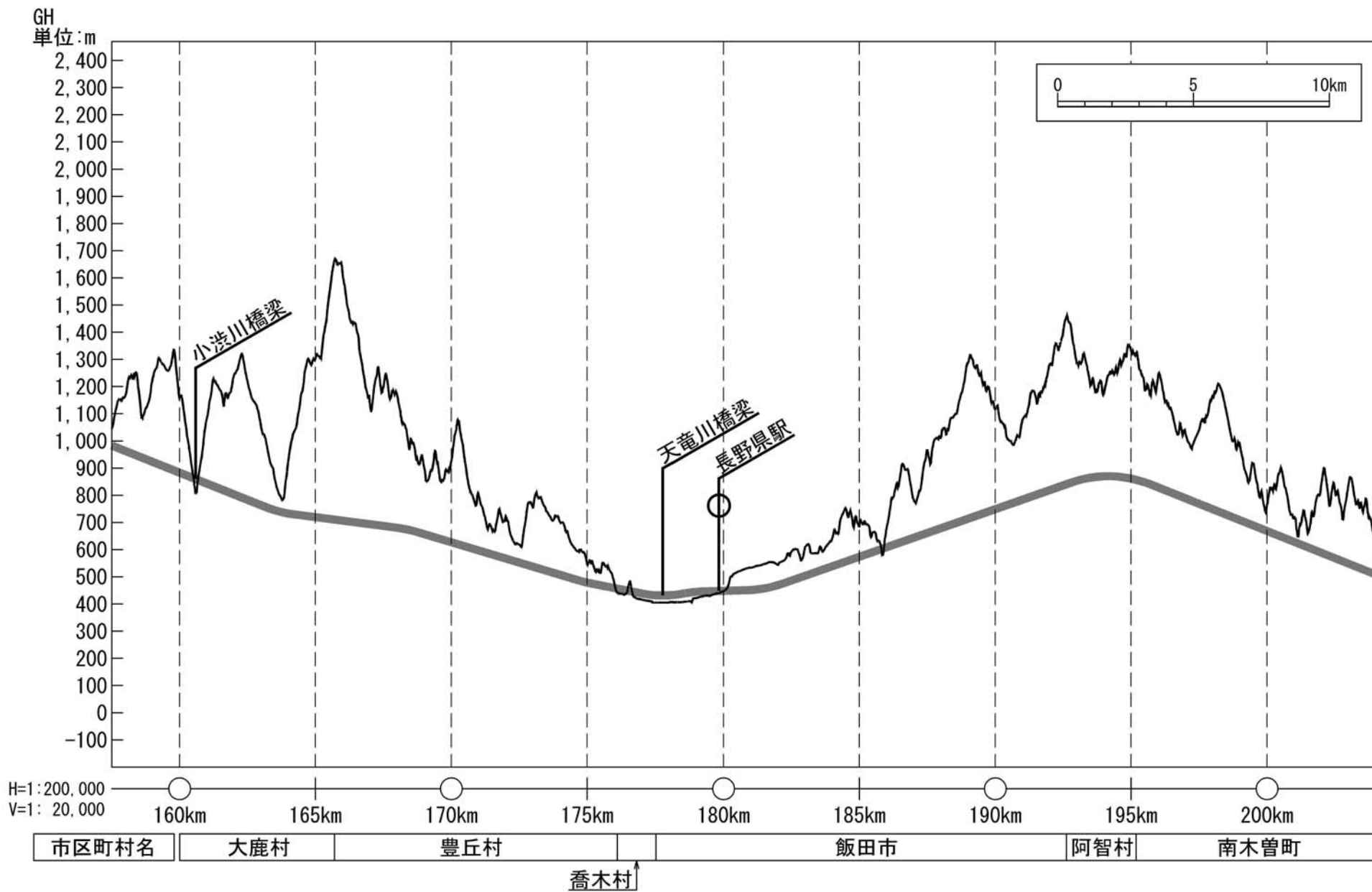
图 2-1(5) 路線概要 (縦断計画)
