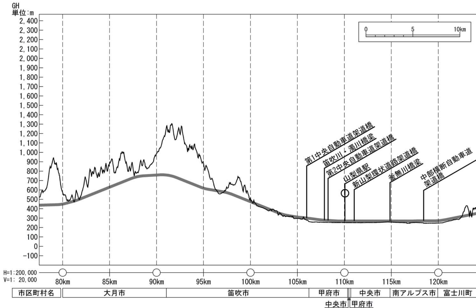
図 2-1(3) 路線概要 (縦断計画)
